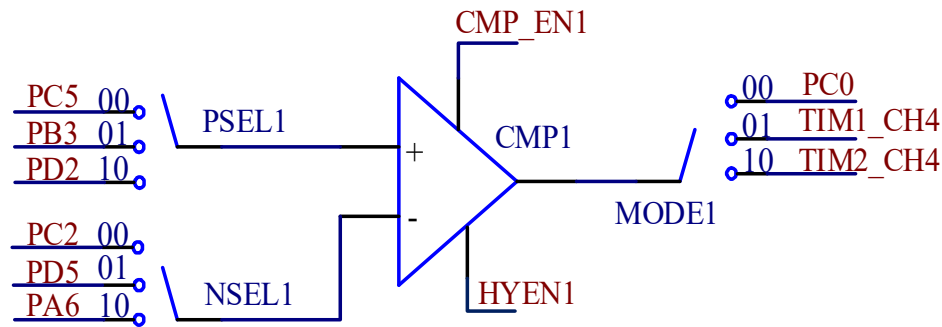
图 17-9 CMP 结构图
