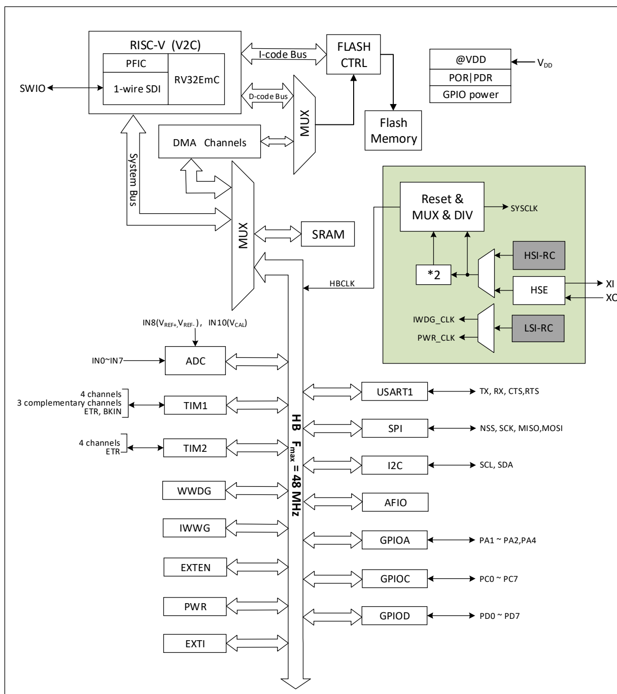
图 1-2 CH32V004 系统框图
