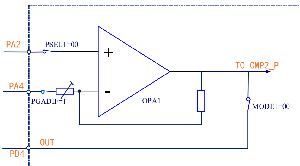
图 17-4 OPA 差分输入示意图
