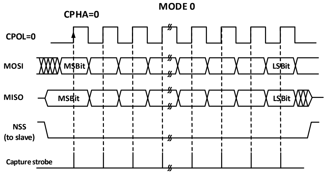
图 16-2 SPI 主模式读写模式 0
