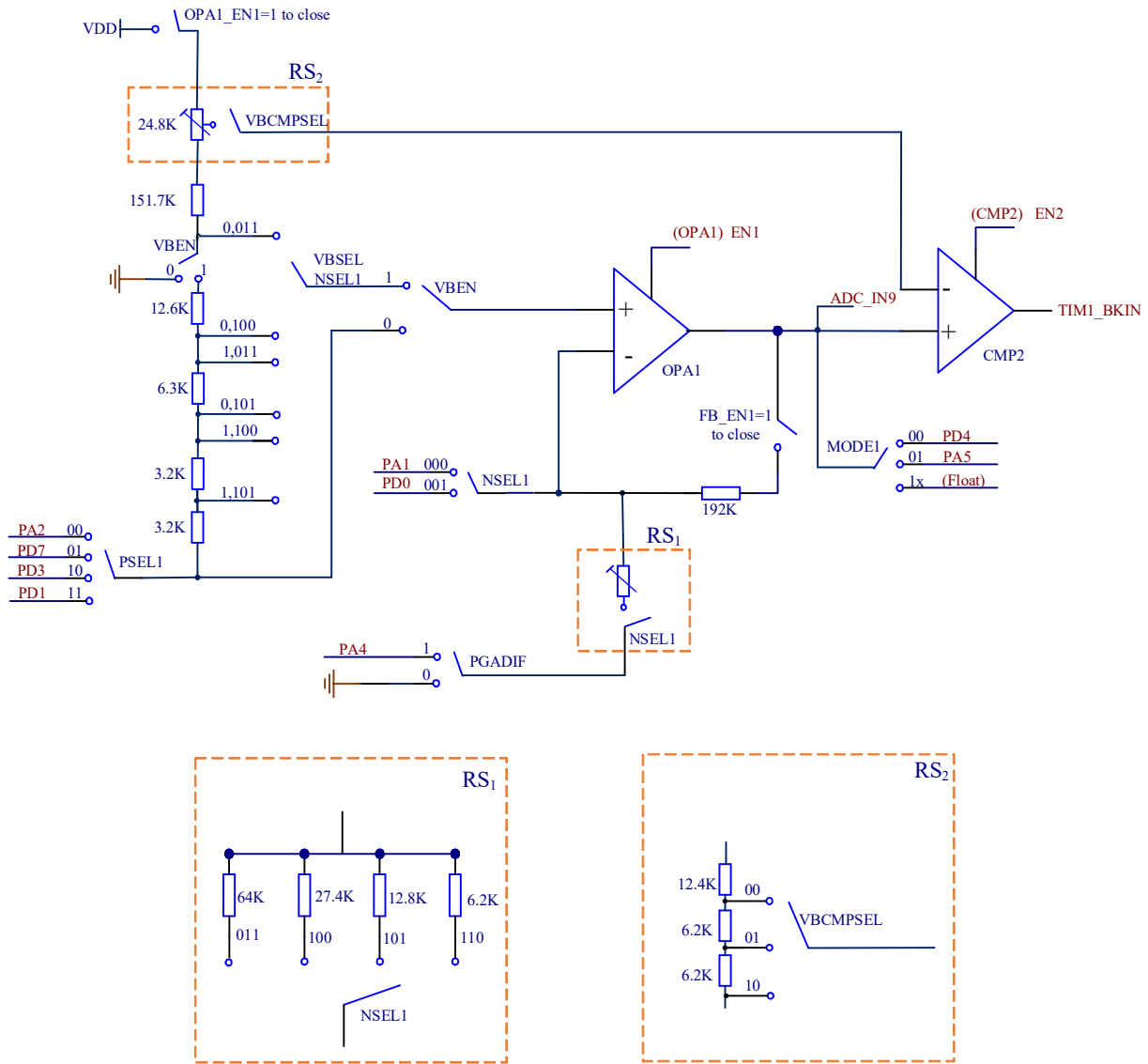
图 17-1 OPA 结构图
