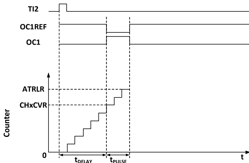
图 11-5 单脉冲的产生
