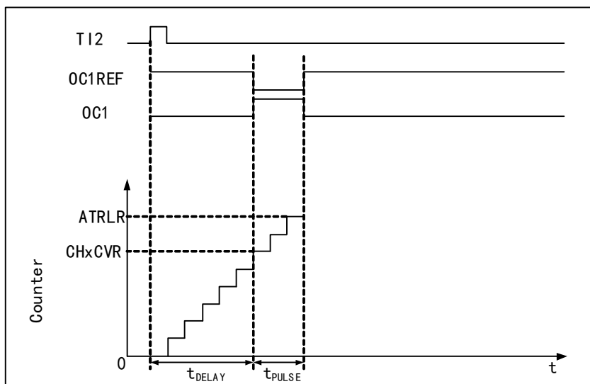
图 12-4 事件产生和脉冲响应
