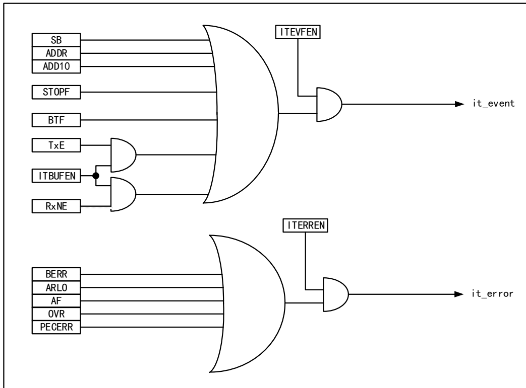
图 15-8 I2C 中断请求
