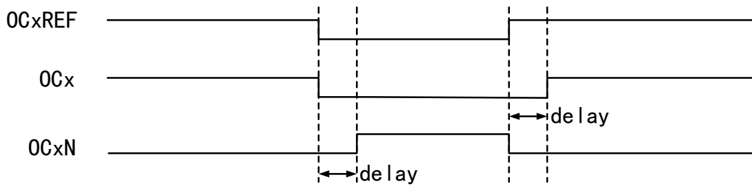
图 11-4 互补输出和死区
