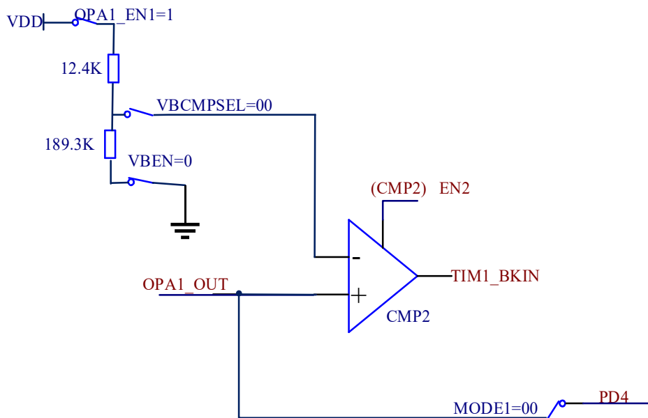
图 17-6 CMP2 独立偏置模式示意图
