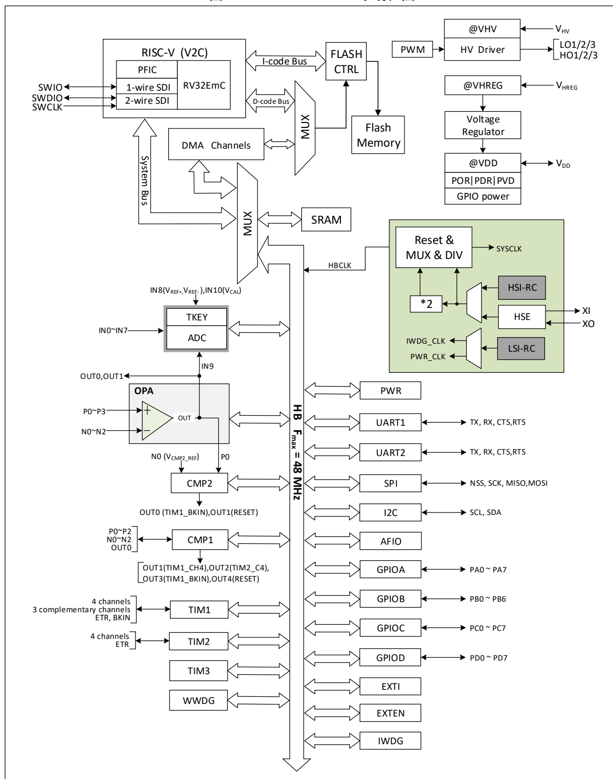
图 1-5-2 CH32M007E8U6 系统框图
