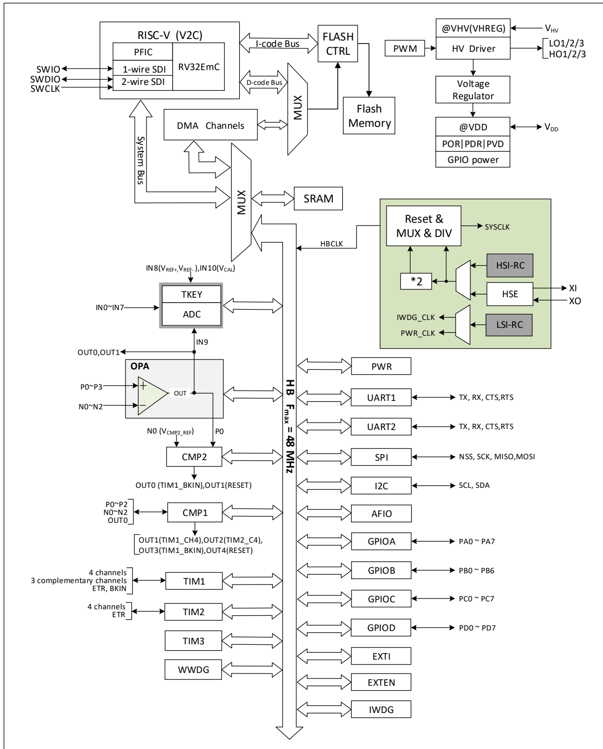
图 1-5-3 CH32M007E8R6 系统框图
