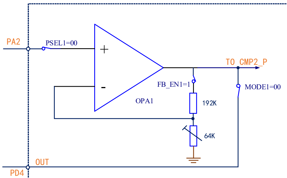
图 17-3 OPA 内部可编程 PGA 示意图
