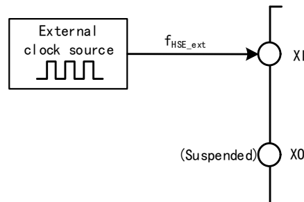
图 3-6 高速时钟源电路
