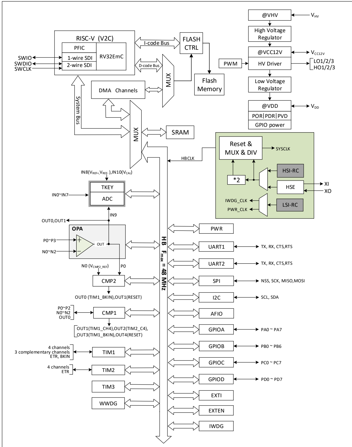
图 1-5-1 CH32M007G8R6 系统框图
