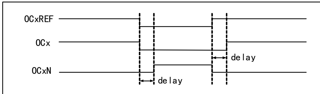
图 9-4 互补输出和死区
