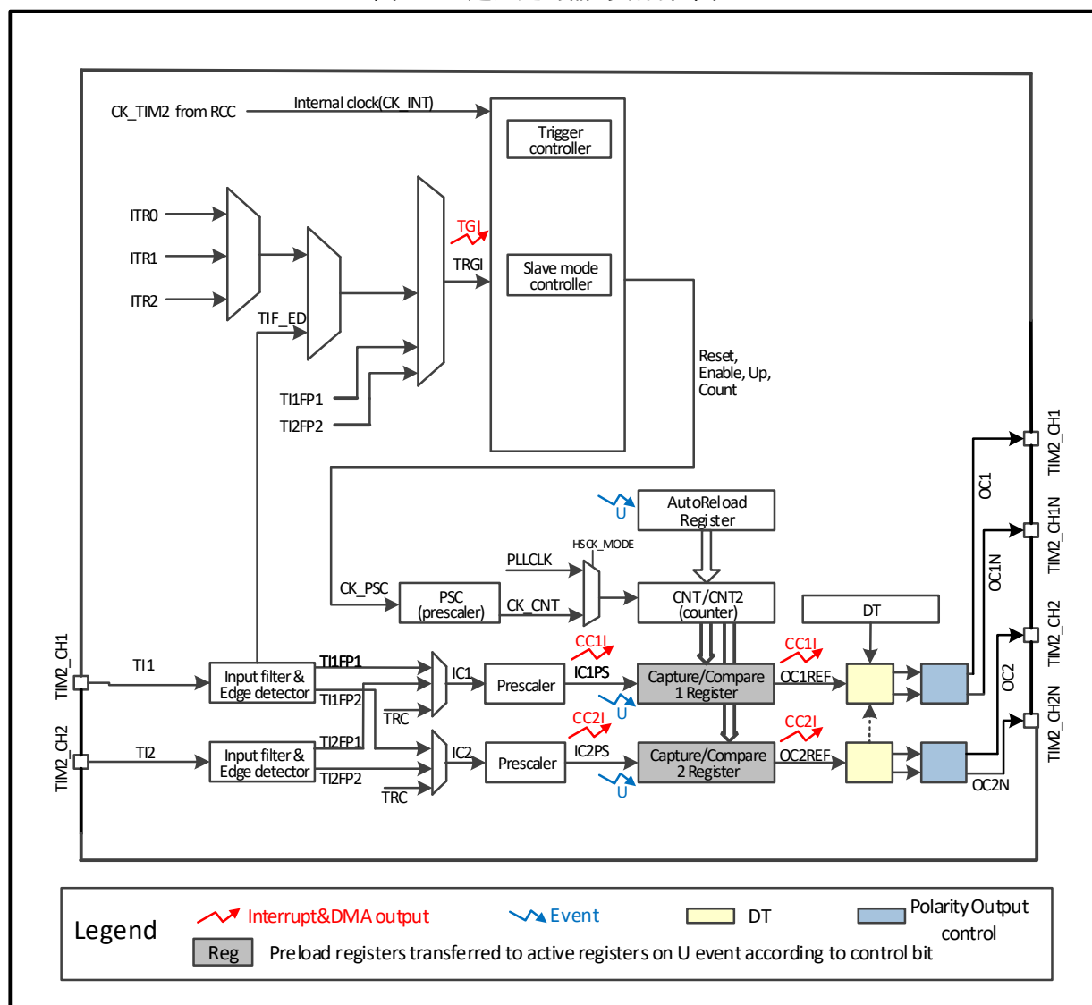
图 10-1 通用定时器的结构框图
