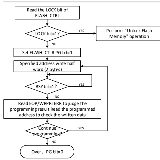
图 14-1 FLASH 编程
