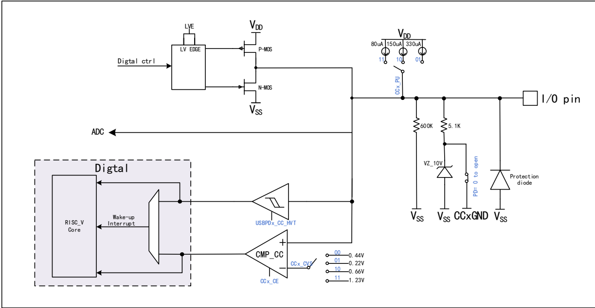
图 15-1 CC 端口结构图
