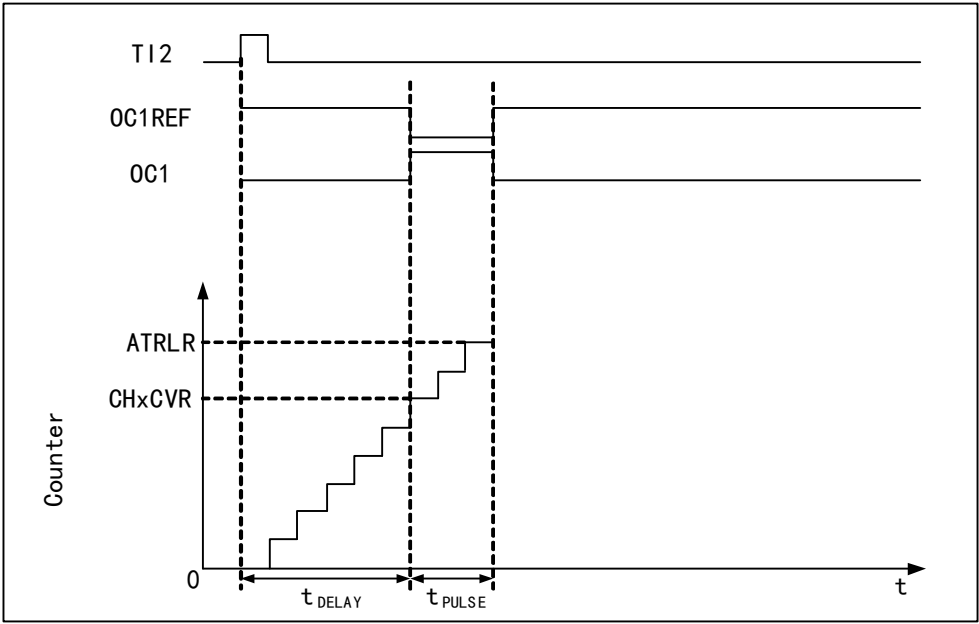
图 10-4 事件产生和脉冲响应
