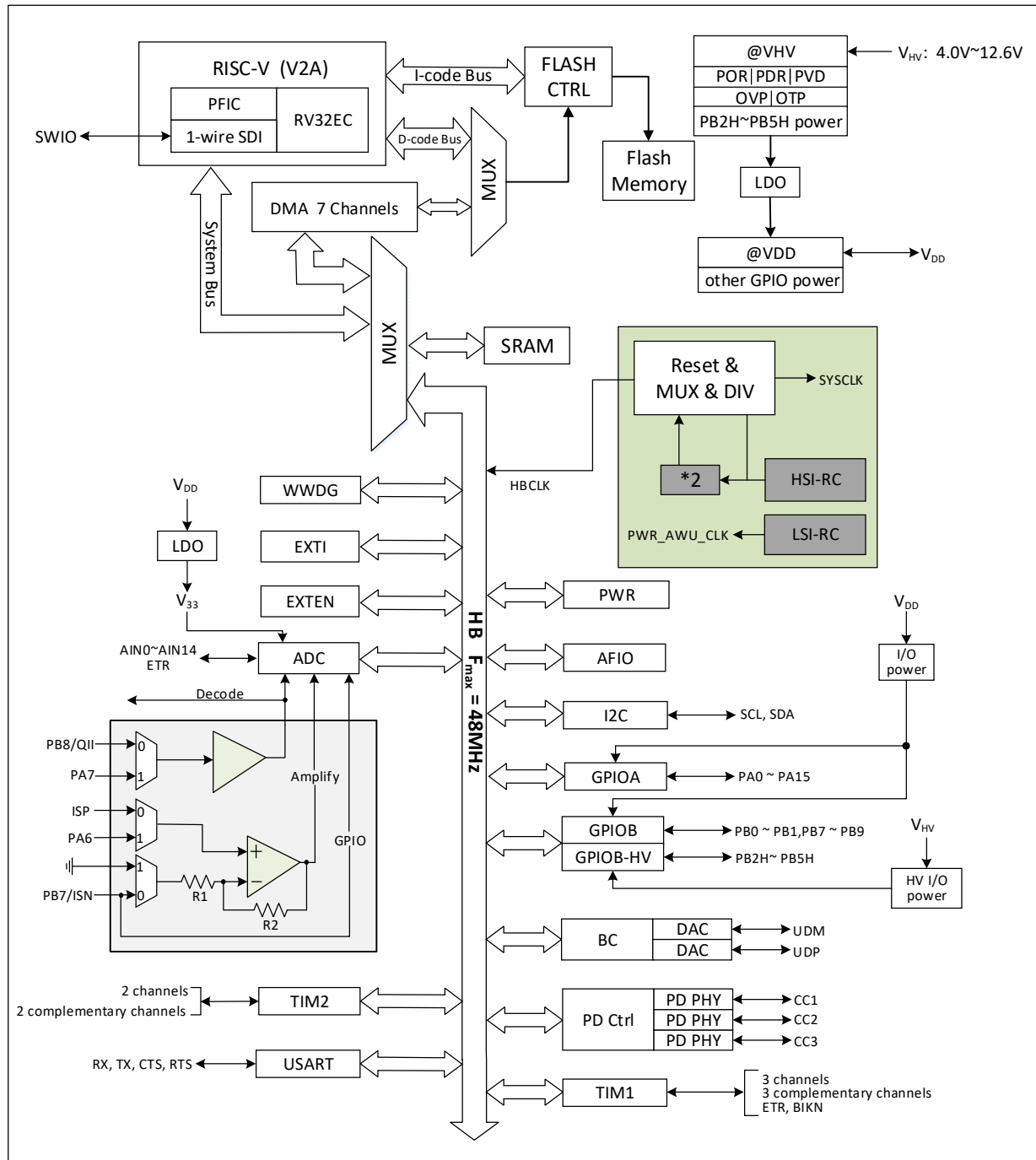
图 1-1 CH641 系统框图
