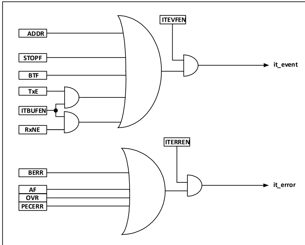
图 12-5 I2C 中断请求
