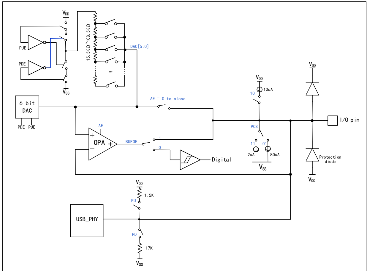
图 16-1 BC 接口结构图
