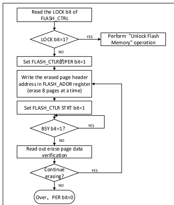
图 14-2 FLASH 页擦除
