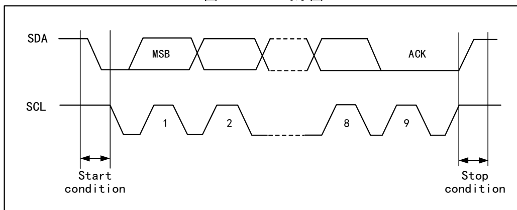
图 12-1 I2C 时序图
