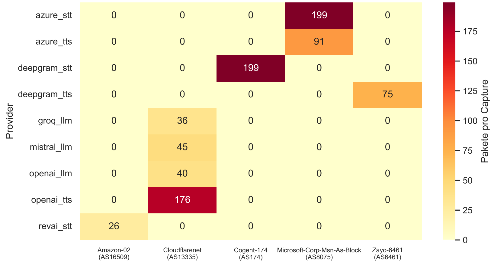
Jeder Provider kontaktiert genau 1 ASN (0/9 Nebenkommunikation) — 4/9 ueber Cloudflare-Edge
