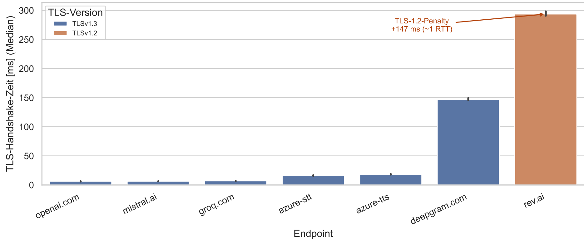
Veraltetes TLS 1.2 kostet Rev.ai +147 ms (~1 RTT) gegenüber TLS 1.3 (n=35/Endpoint, 95%-CI)
