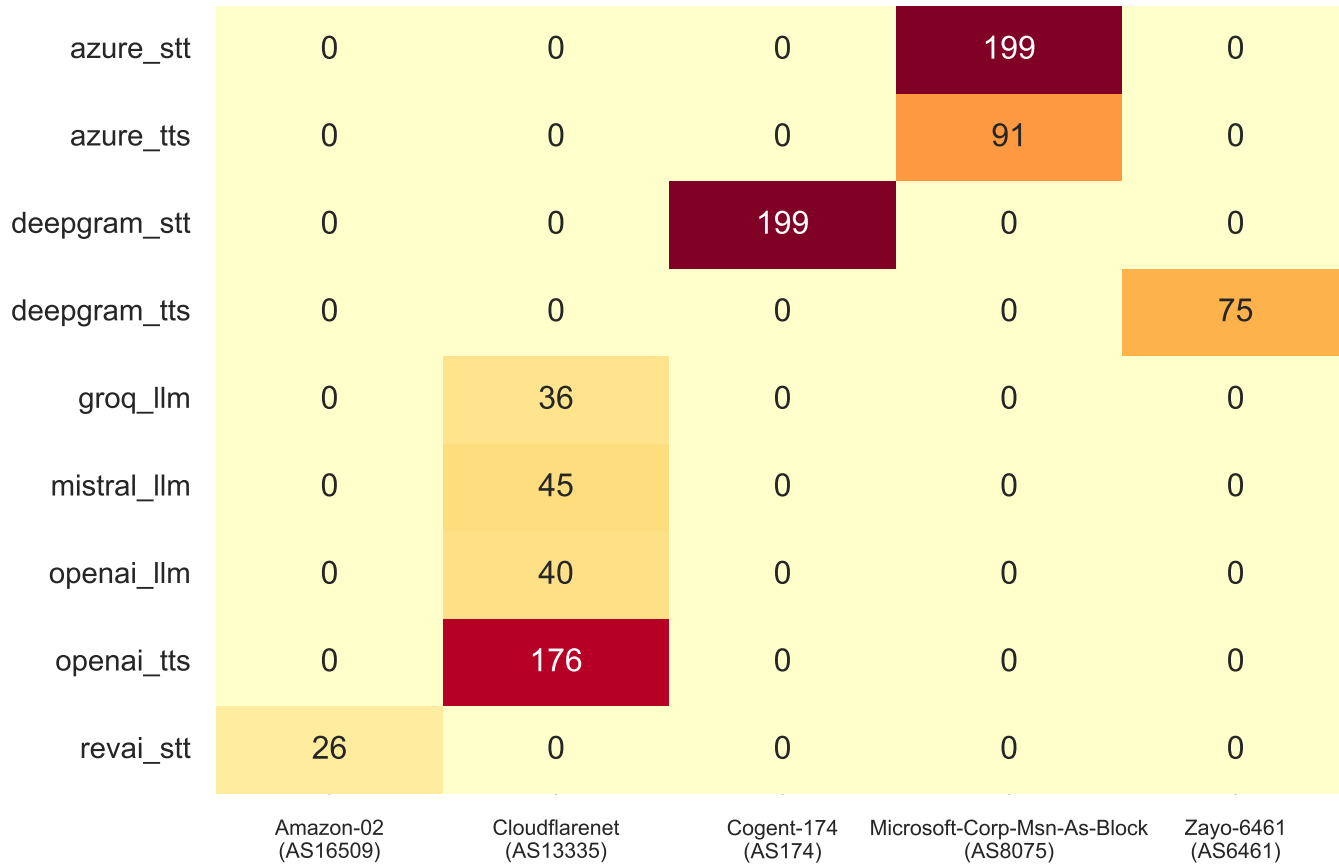
Jeder Provider kontaktiert genau 1 ASN (0/9 Nebenkommunikation) — 4/9 ueber Cloudflare-Edge
