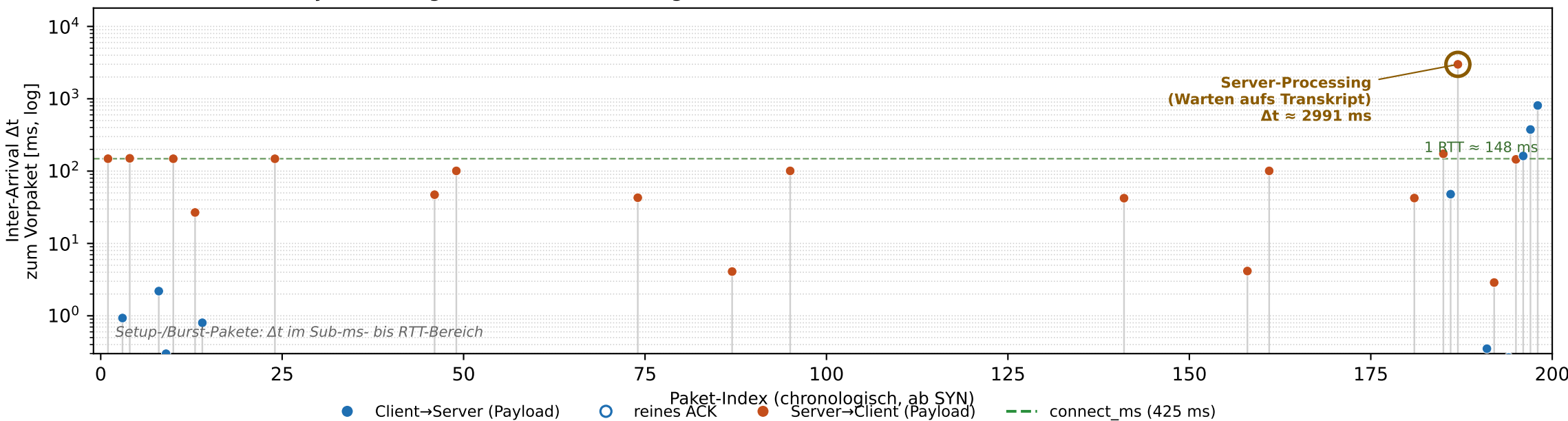
(B) Inter-Arrival-Time je Paket (log): nur Server-Processing als Ausreisser — KEINE Client-Sendelücke
