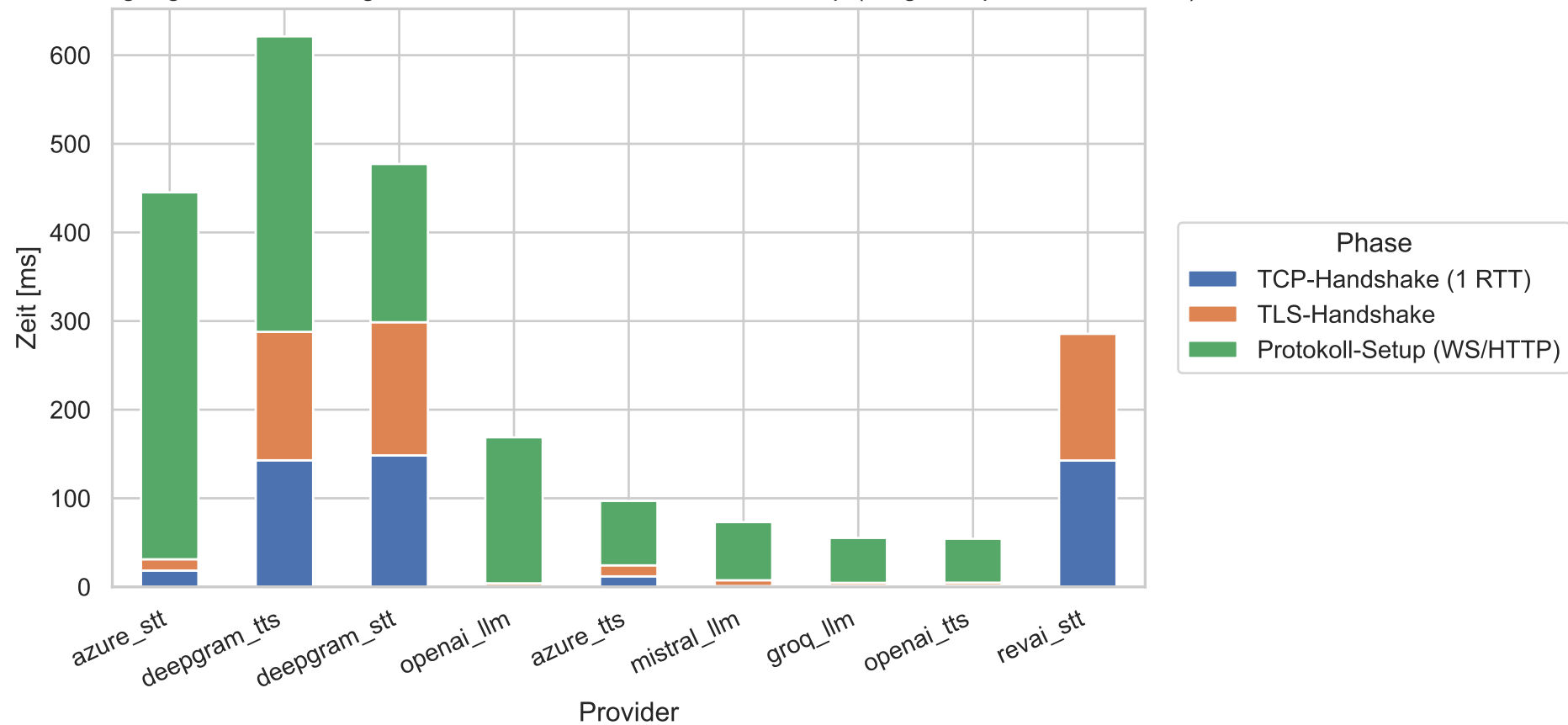
Zerlegung des Verbindungsaufbaus: TCP + TLS + Protokoll-Setup (Single-Capture 2026-06-08)
