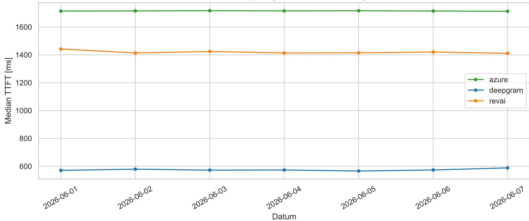
Median TTFT pro Tag - Stabilitaet ueber 7 Tage
