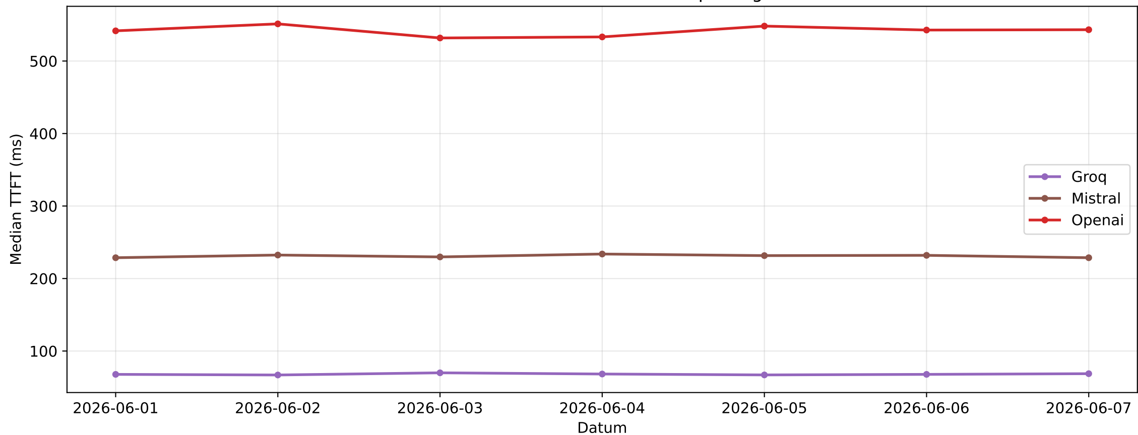
Zeitlicher Drift: Median TTFT pro Tag
