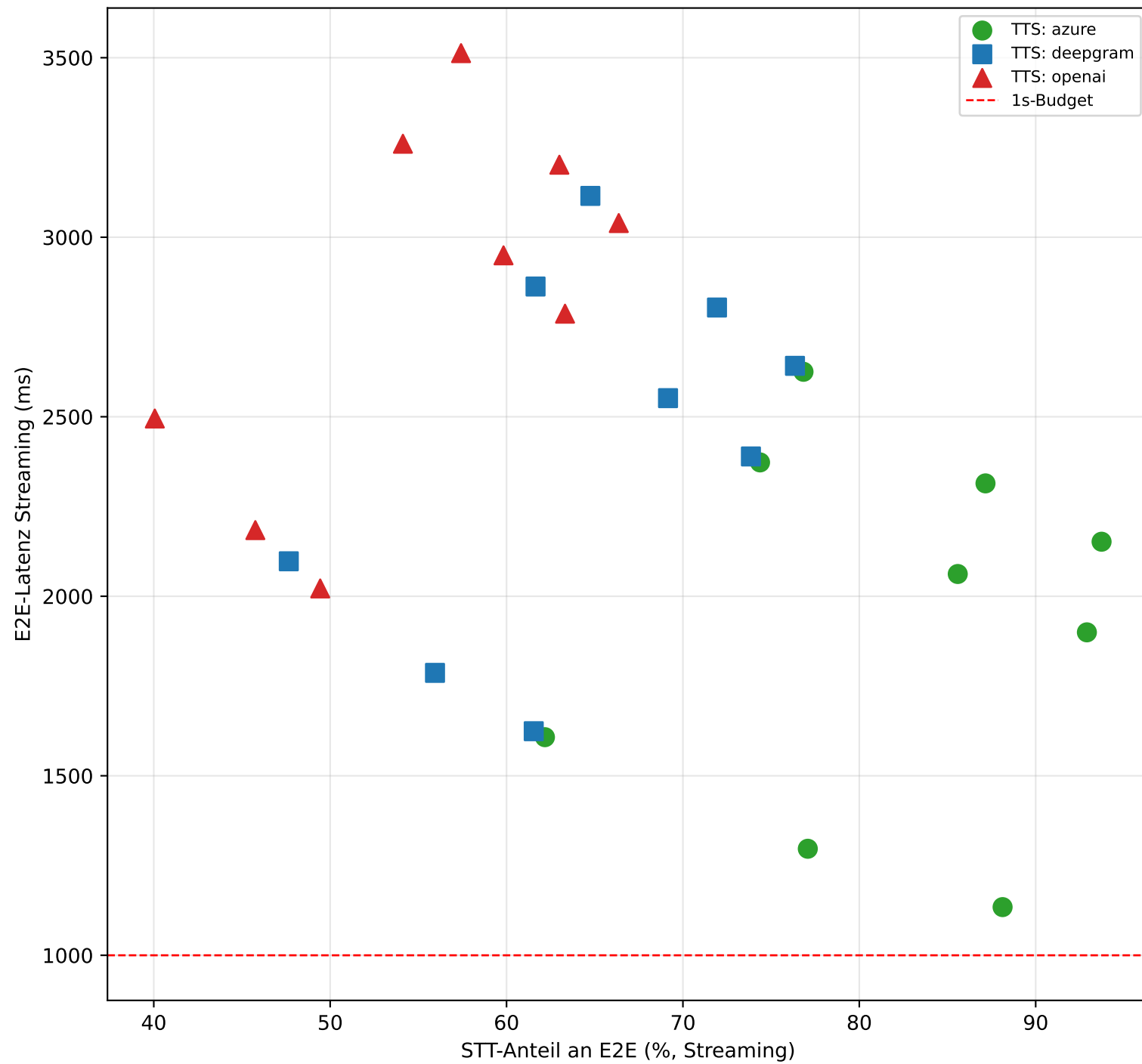
STT-Anteil vs. Gesamt-E2E (Punkte = TTS-Provider)
