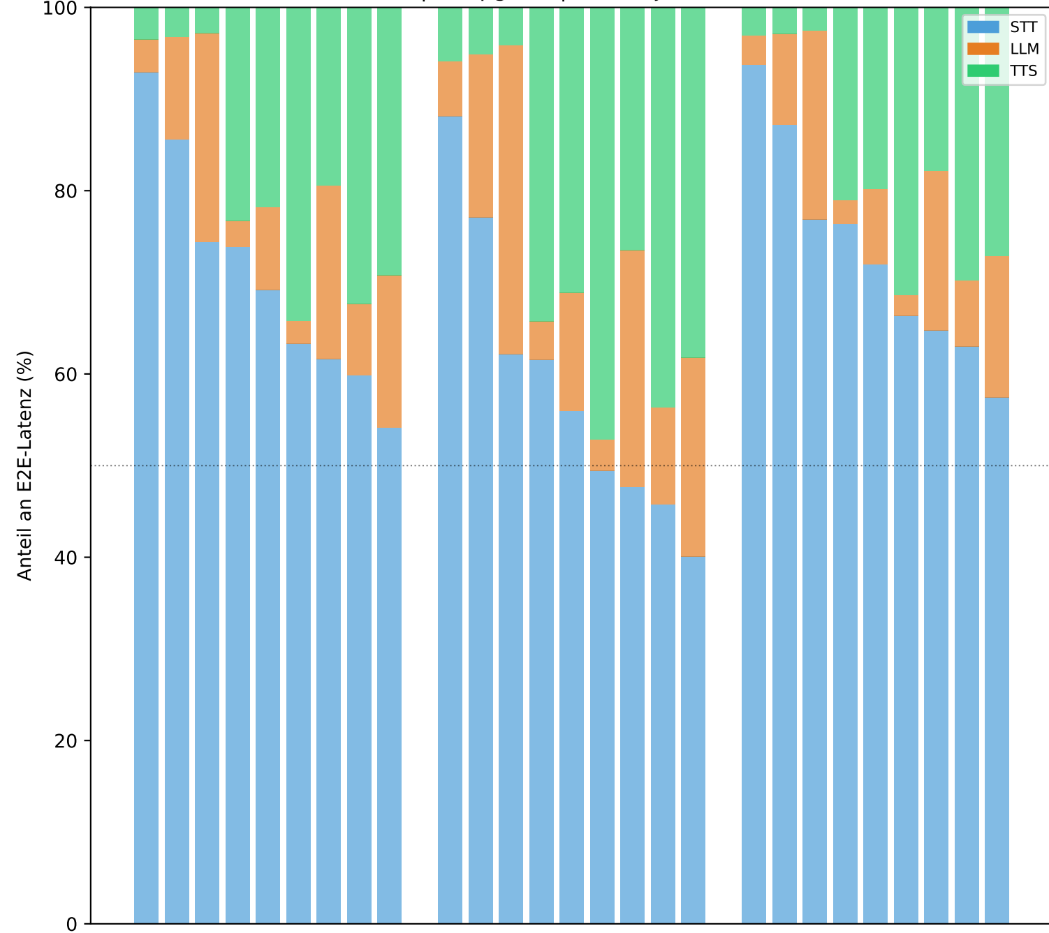
Layer-Anteile pro STT-Gruppe (Azure | Deepgram | Rev.ai, je 9 Combos)
