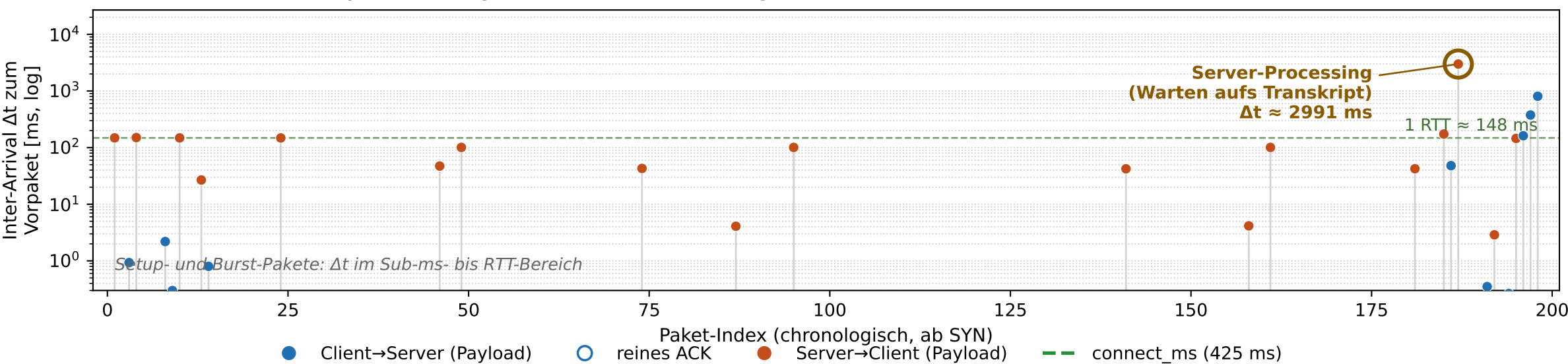
(B) Inter-Arrival-Time je Paket (log): nur Server-Processing als Ausreisser — KEINE Client-Sendelücke
