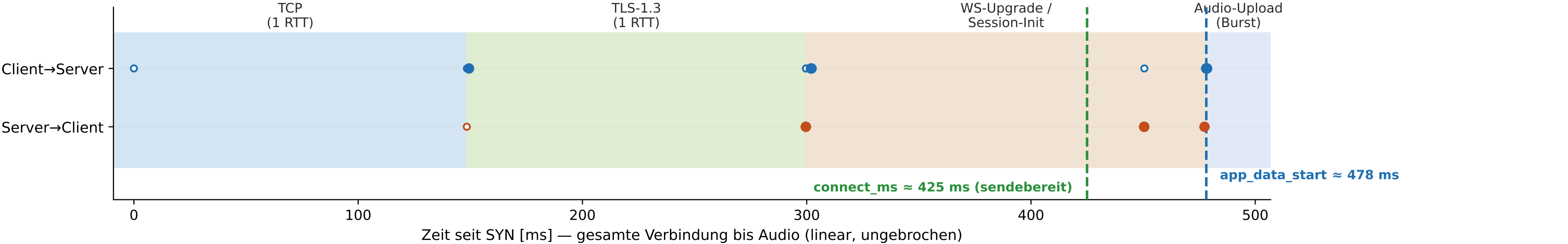
(A2) Lückenloser, RTT-dominierter Aufbau — jede Pause ist eine RTT, KEINE Client-Wartezeit
