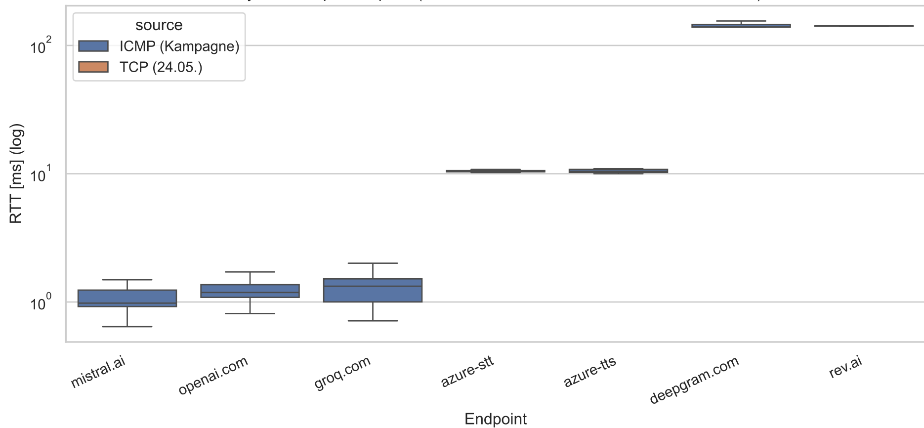
Layer-1-RTT pro Endpoint (sortiert nach Median, n=91-182 ICMP + 10 TCP)
