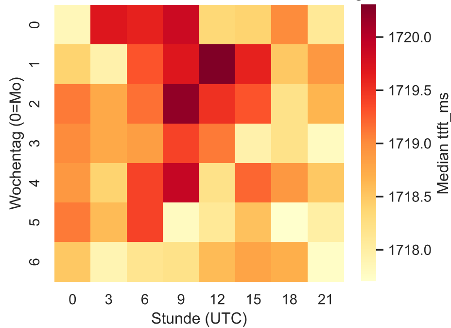
azure: Median TTFT nach Stunde × Wochentag
