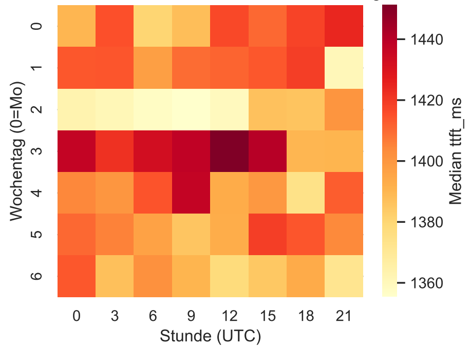
revai: Median TTFT nach Stunde × Wochentag
