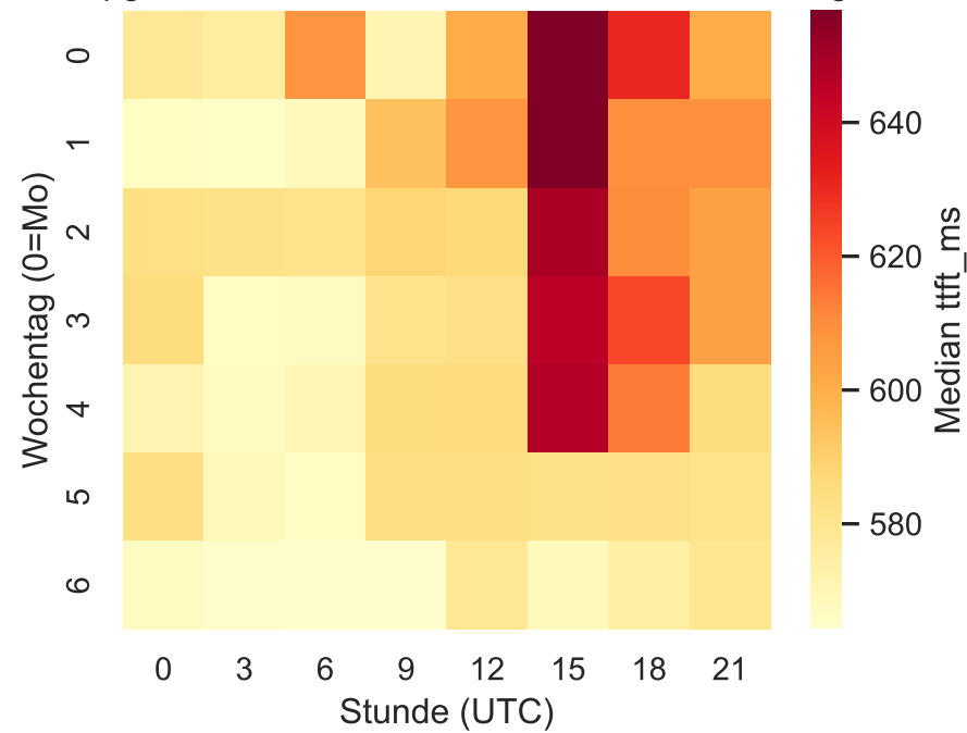
deepgram: Median TTFT nach Stunde × Wochentag
