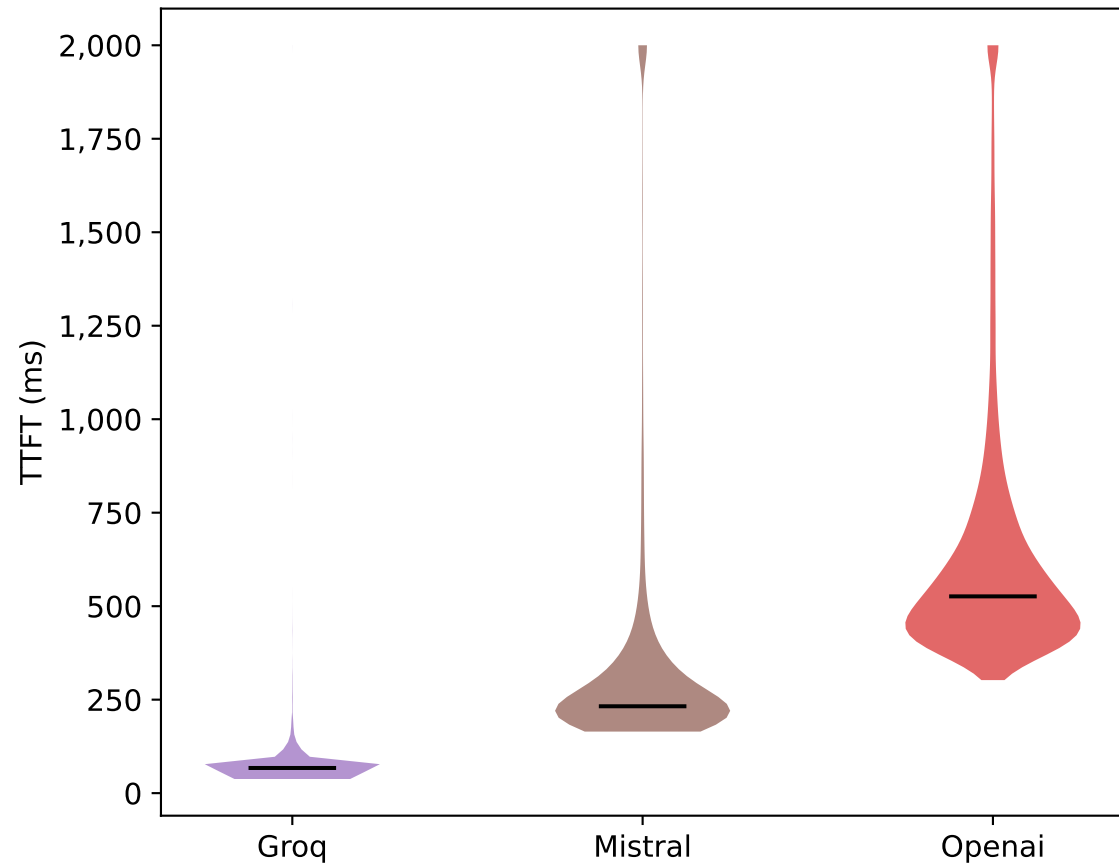
Verteilung TTFT (Werte > 2 s abgeschnitten)
