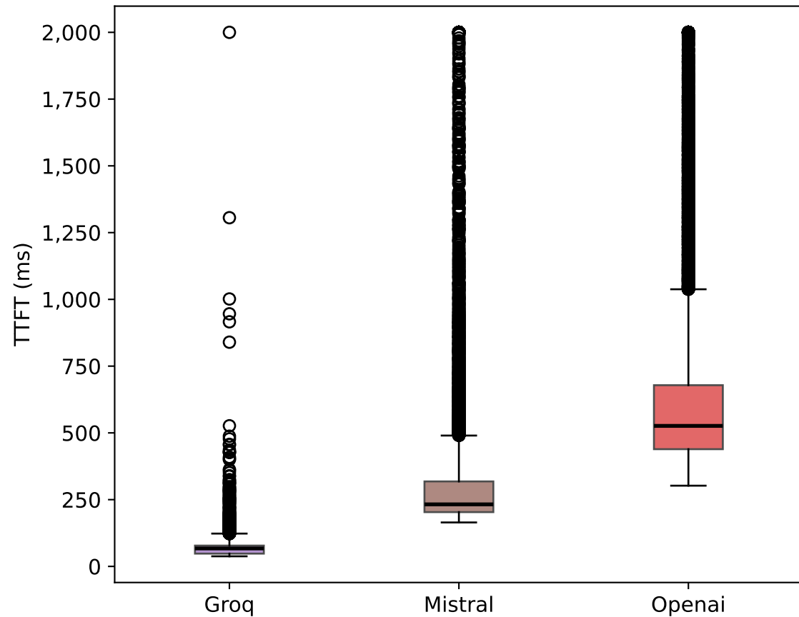
Box-Plot TTFT (Werte > 2 s abgeschnitten)
