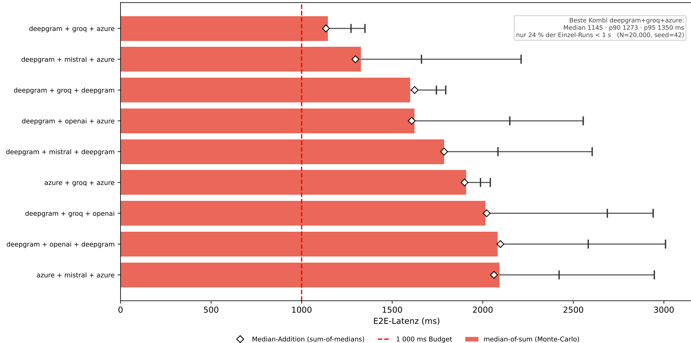
Monte-Carlo-Validierung (Top-9): median-of-sum \approx Median-Addition ( \Delta < 2\% ), Whisker = p90/p95 — die Streuung, nicht der Median, entscheidet das 1-s-Budget
