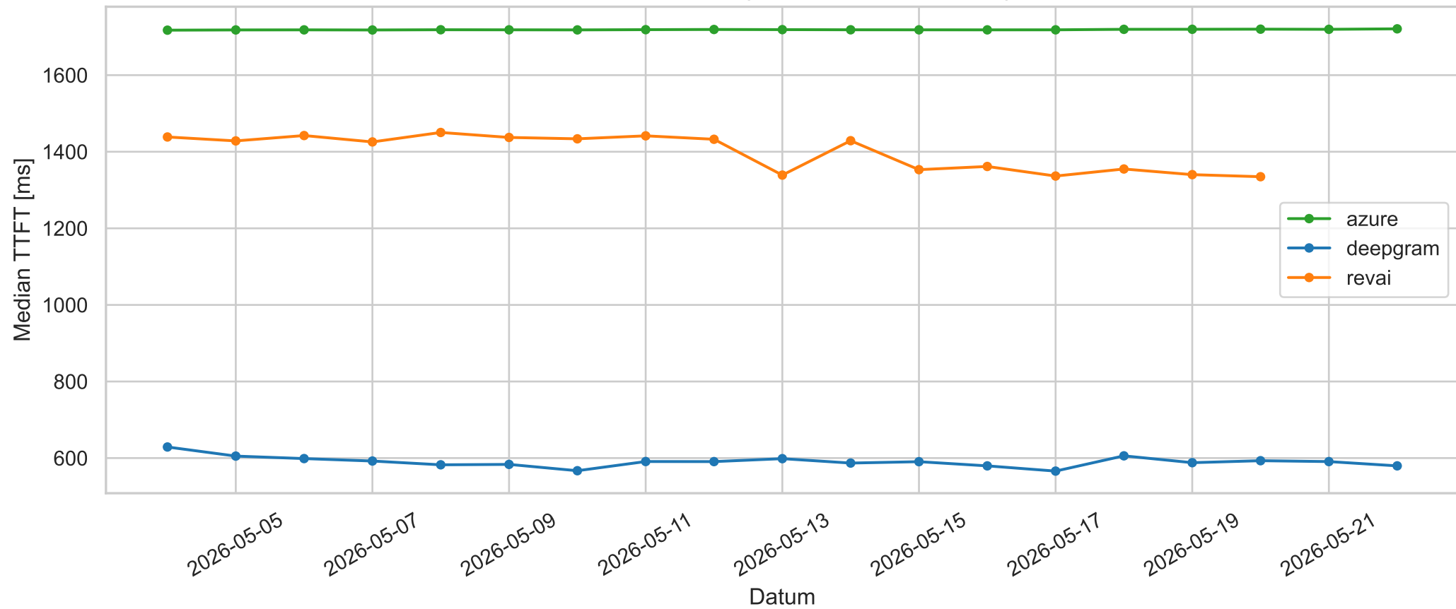
Median TTFT pro Tag - Stabilität ueber 18 Tage
