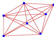
dense
