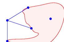
implicit
