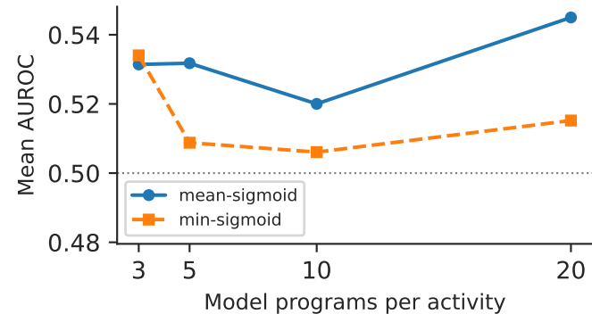
HumanAct12
