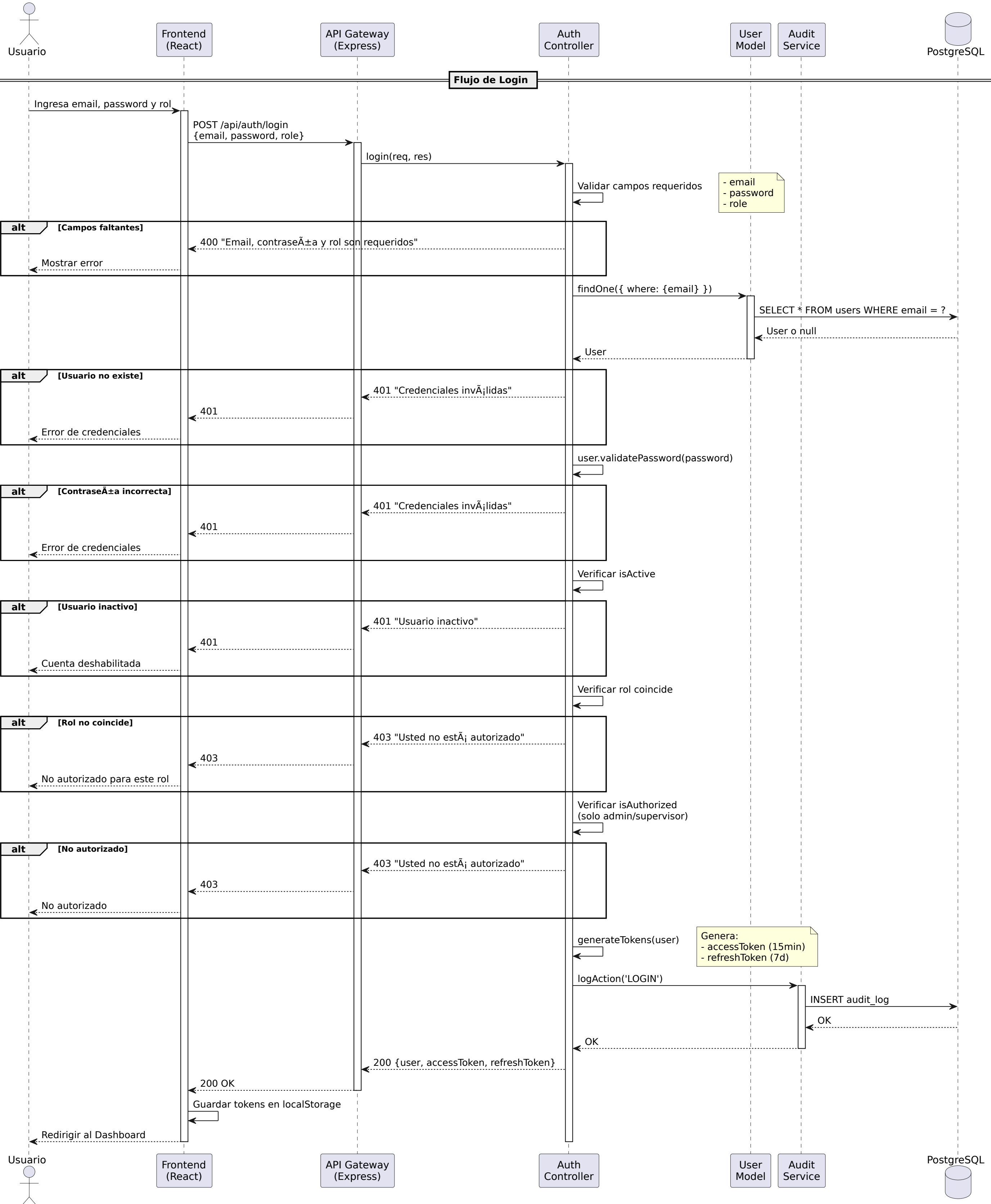
Diagrama de Secuencia - Login de Usuario
