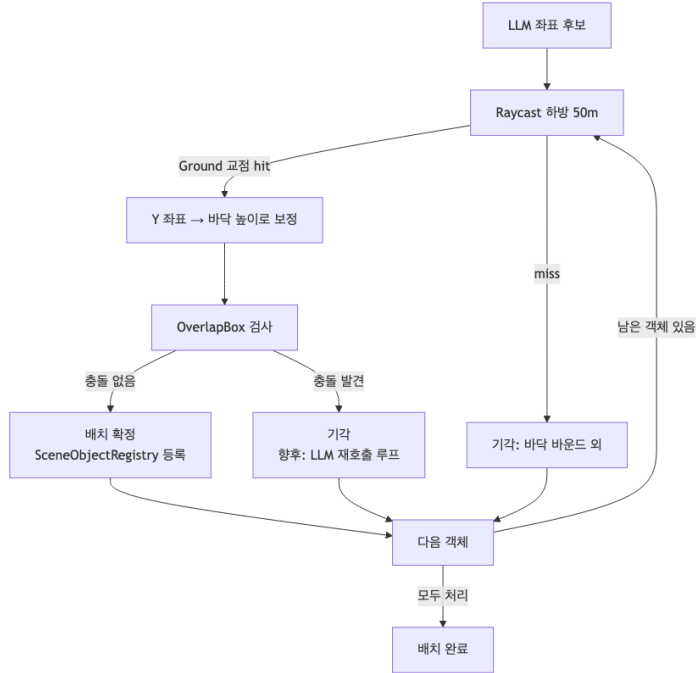
그림 2. LayoutValidator의 Raycast → Snap → OverlapBox 검증 루프.
