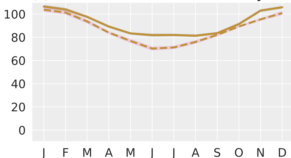
(d) Low cloud cover
