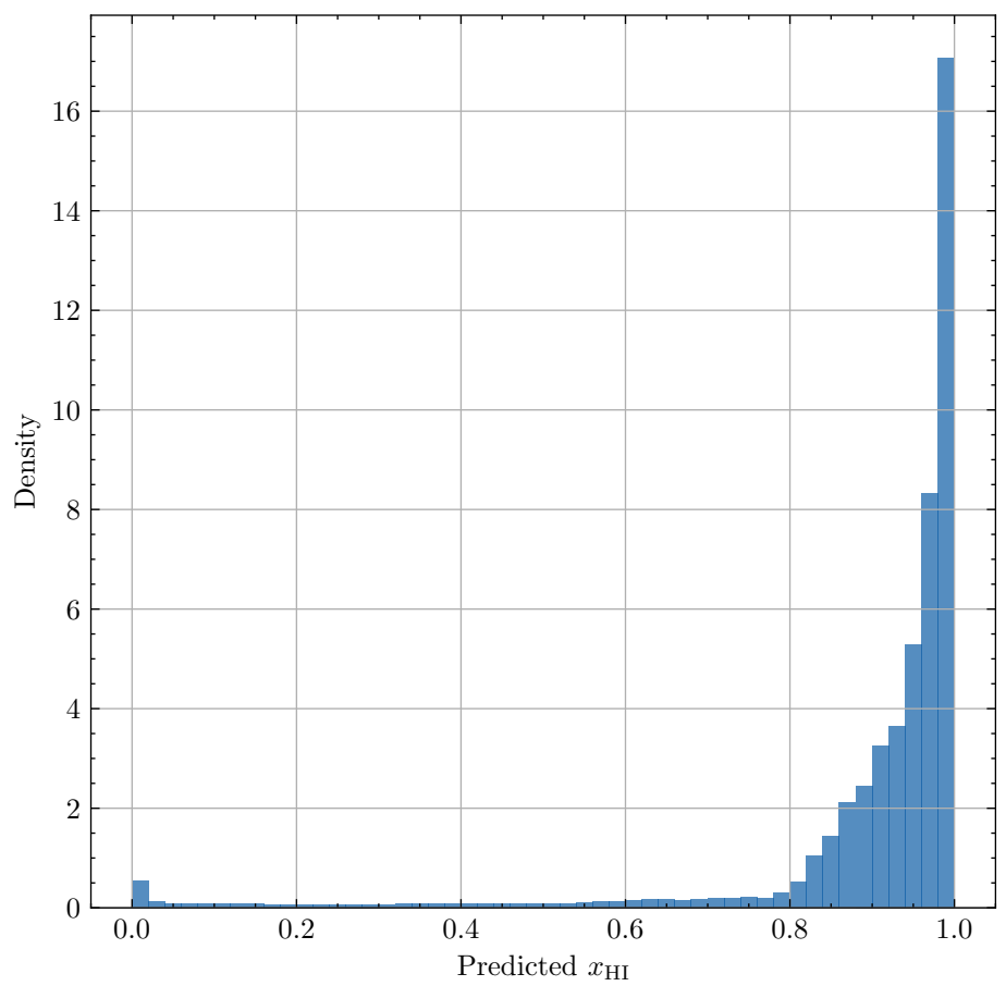
Redshift z = 12.24
