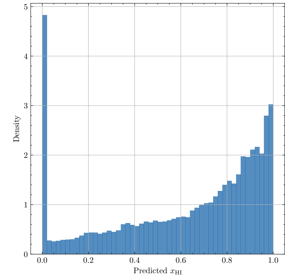
Redshift z = 11.21
