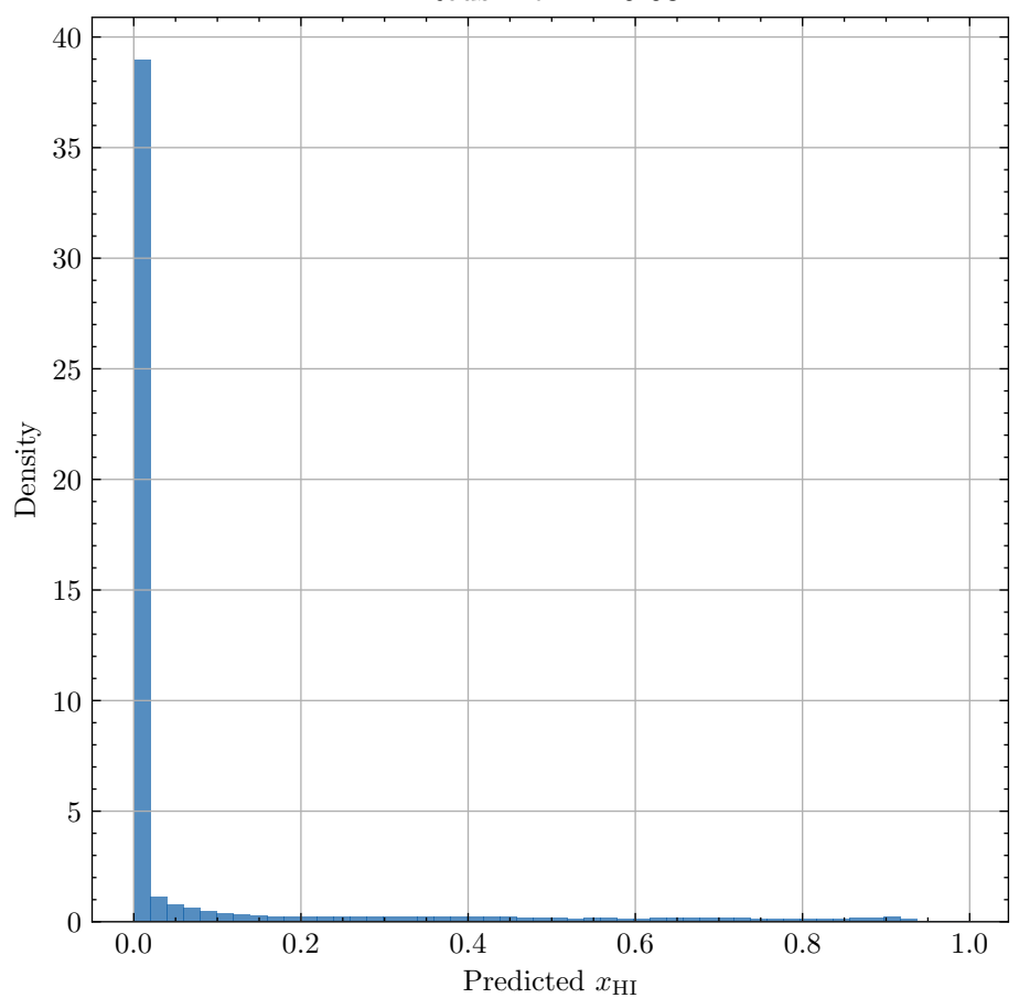
Redshift z = 7.59
