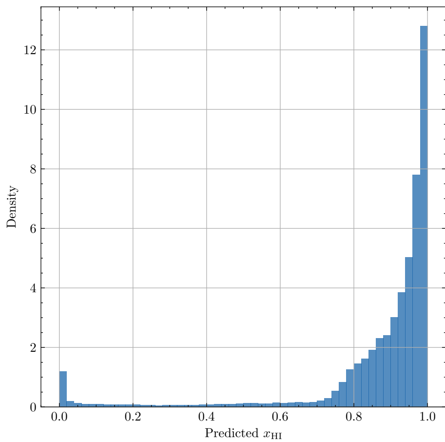
Redshift z = 11.72
