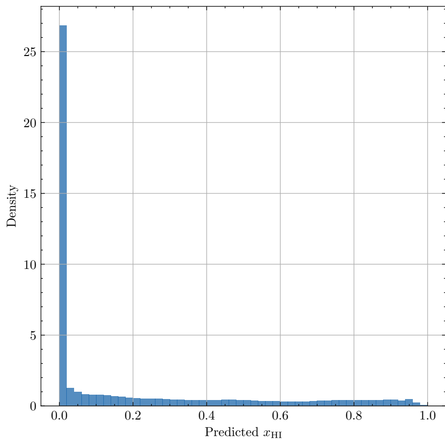
Redshift z = 8.62
