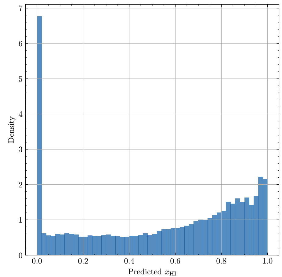
Redshift z = 10.69
