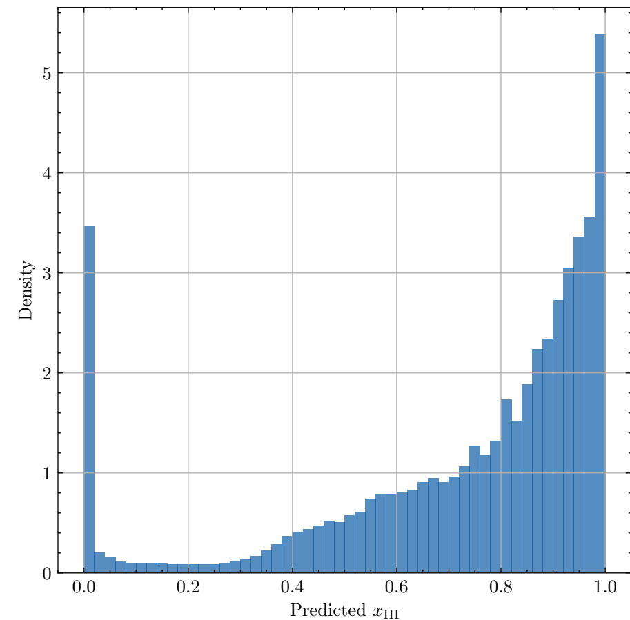
Redshift z = 11.72
