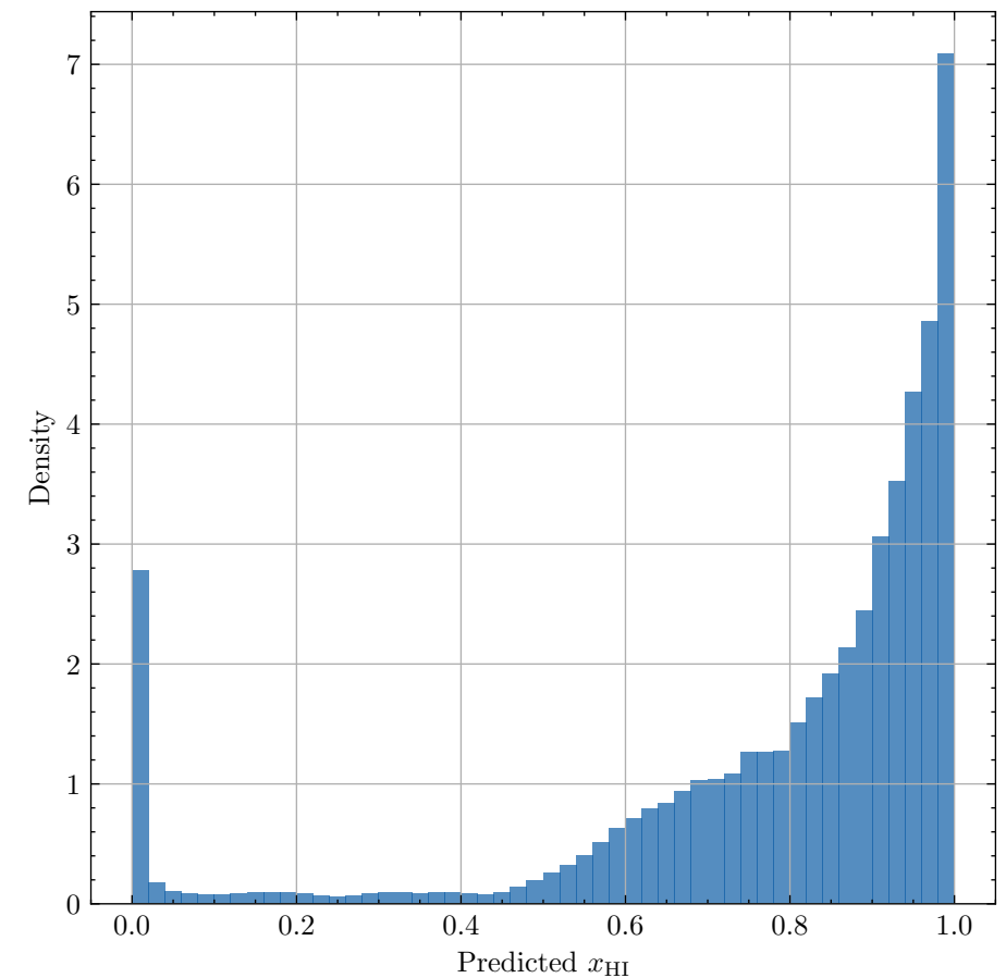
Redshift z = 12.24
