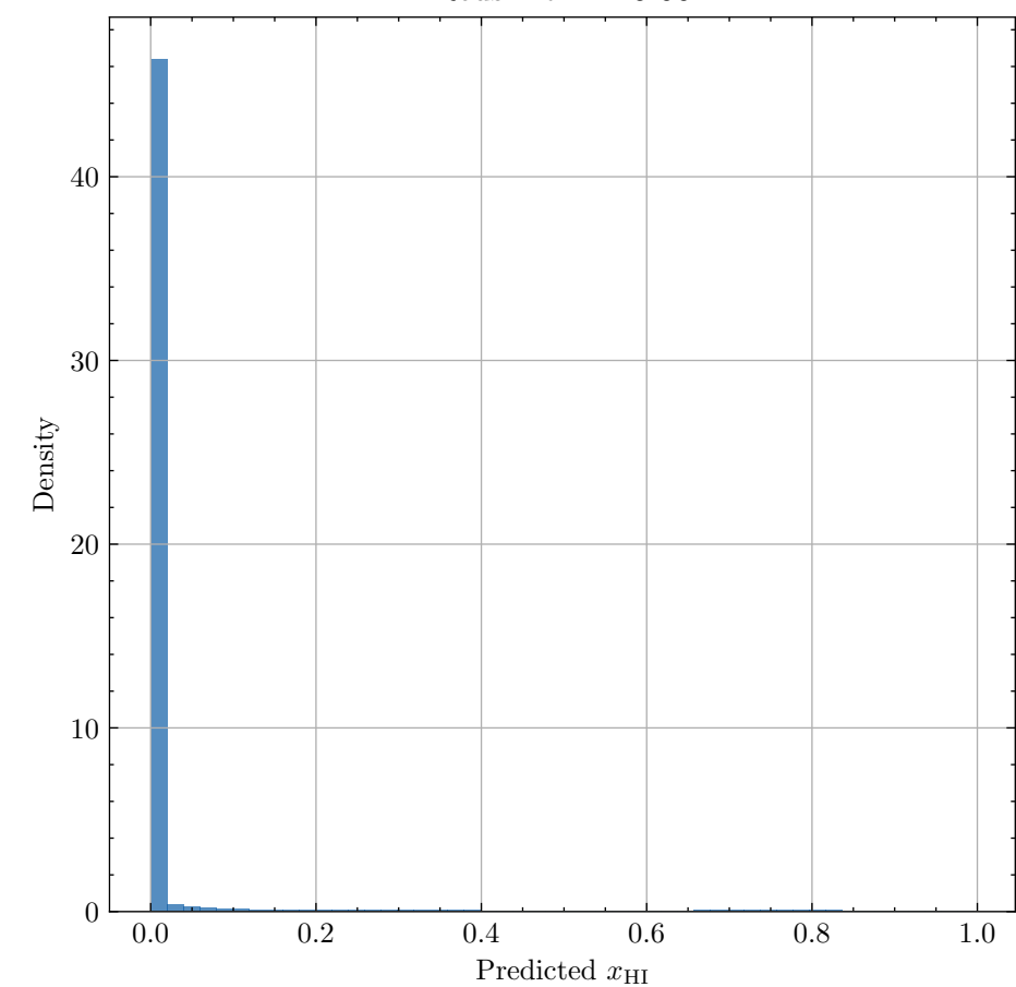
Redshift z = 6.55
