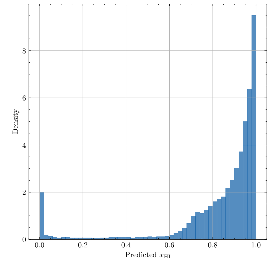
Redshift z = 11.21
