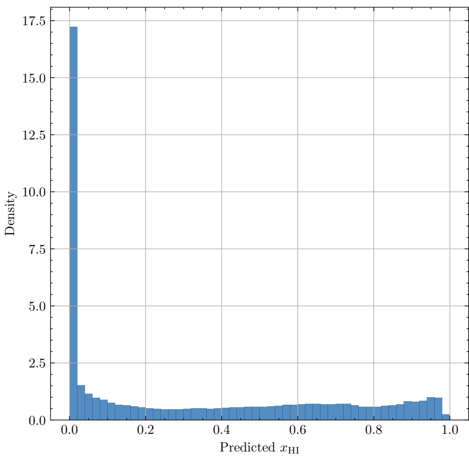
Redshift z = 9.66
