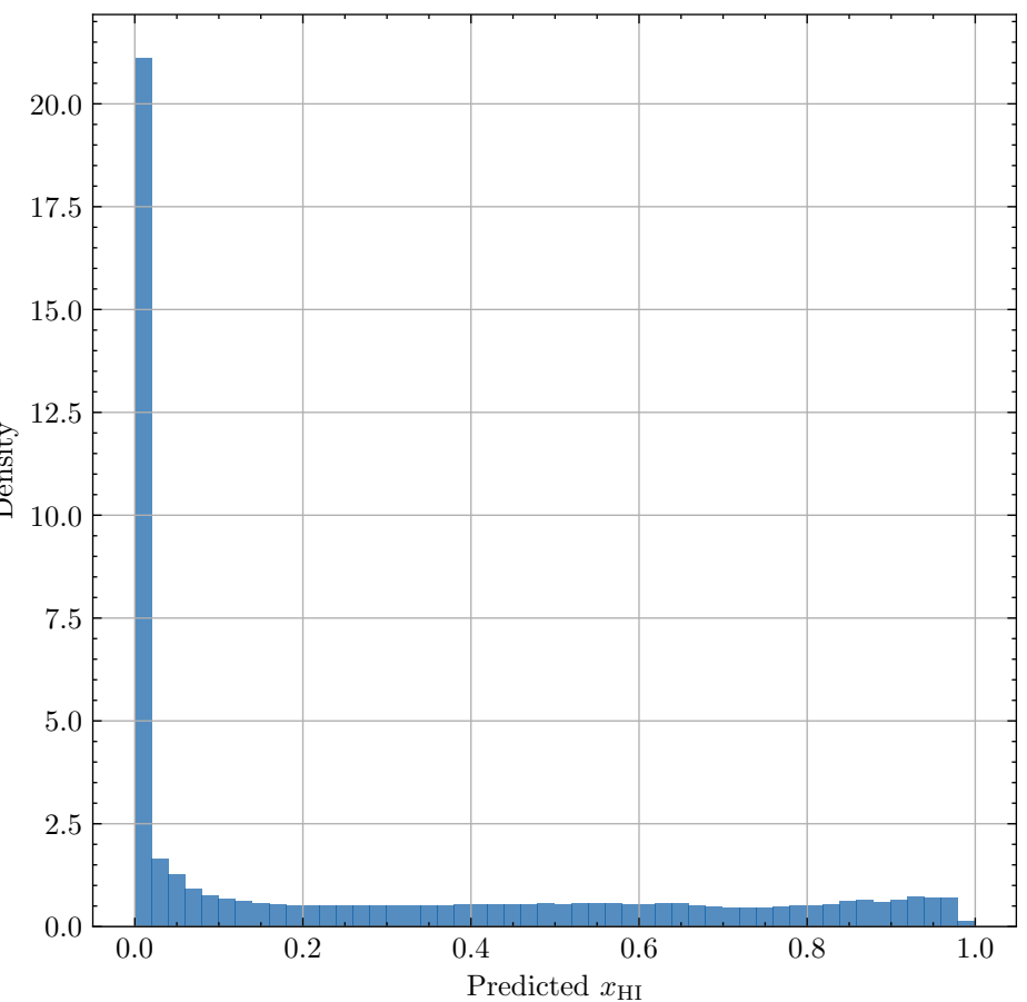
Redshift z = 9.14
