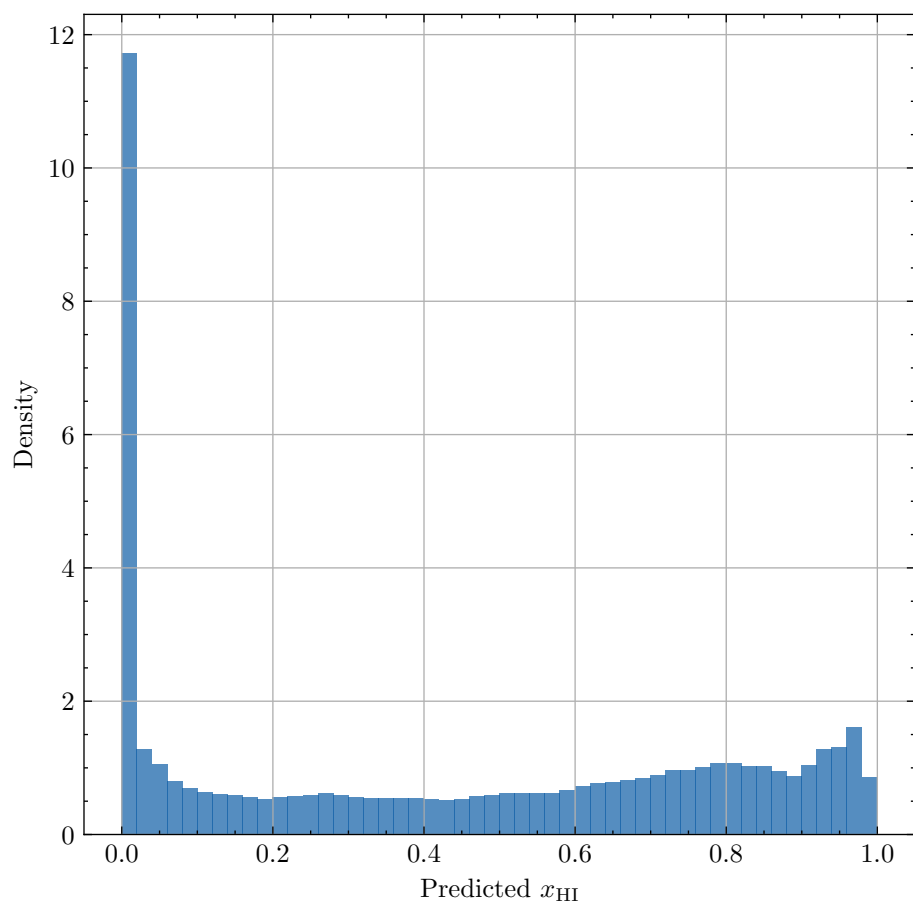
Redshift z = 10.17
