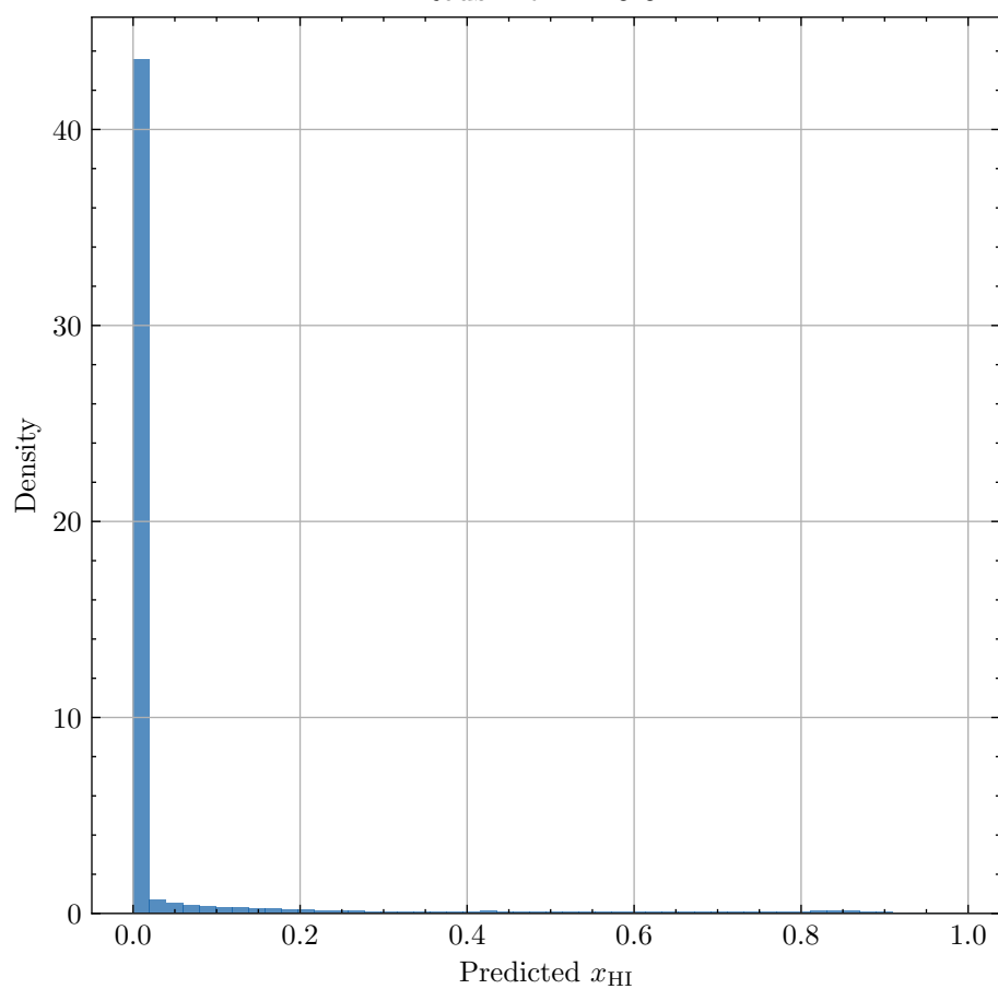
Redshift z = 7.07
