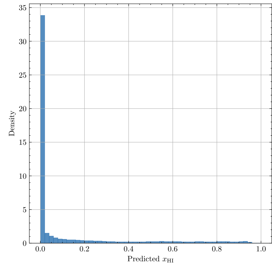
Redshift z = 8.10
