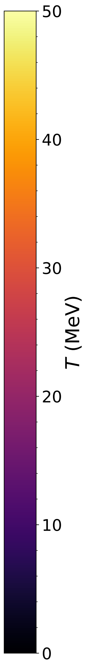
EOS-V 1.3 M_{\odot} - 1.3 M_{\odot} t = t_{\text{mrg}} + 3 \text{ ms}
