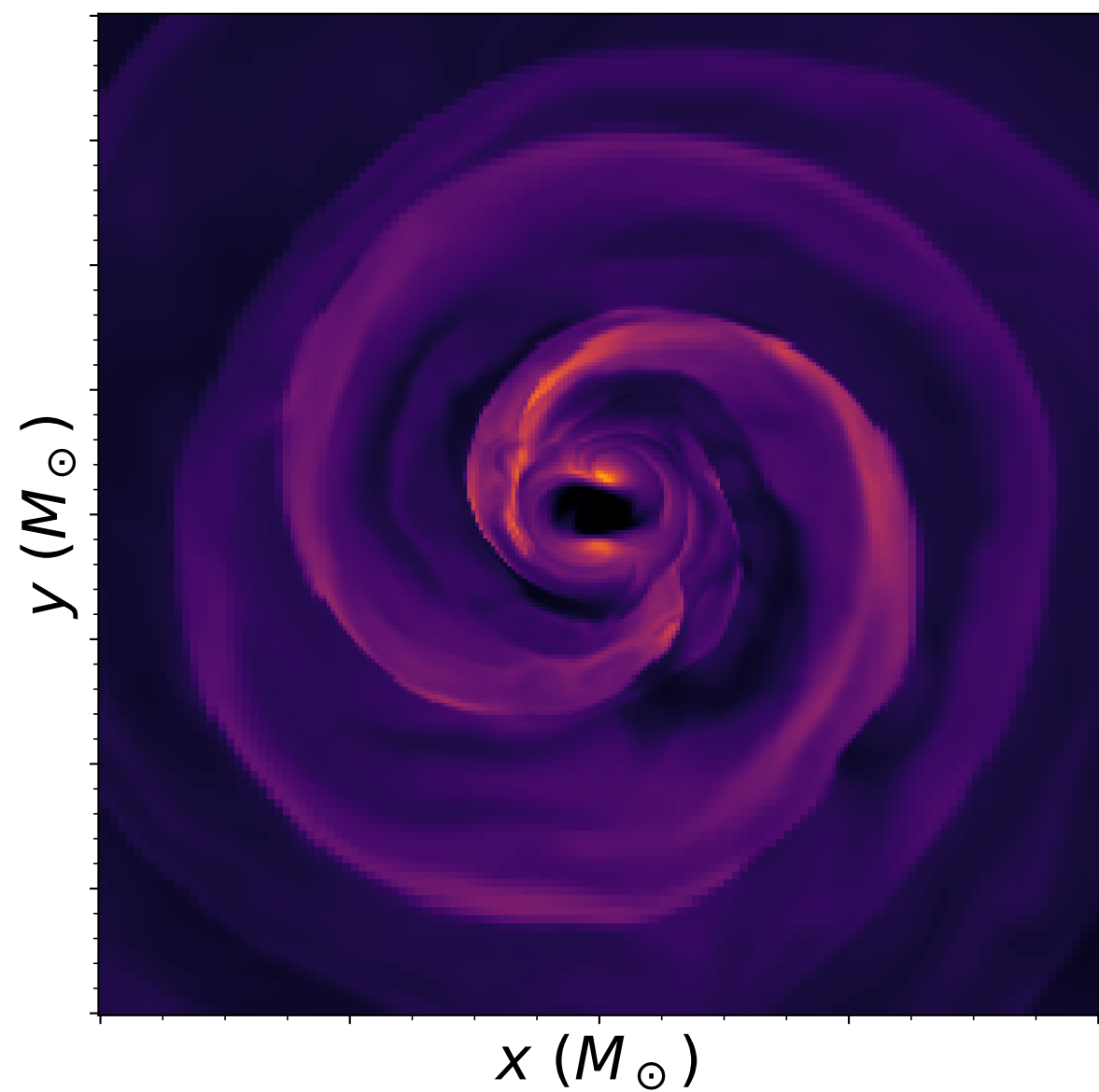
EOS-II 1.3 M_{\odot} - 1.3 M_{\odot} t = t_{\text{mrg}} + 3 \text{ ms}
