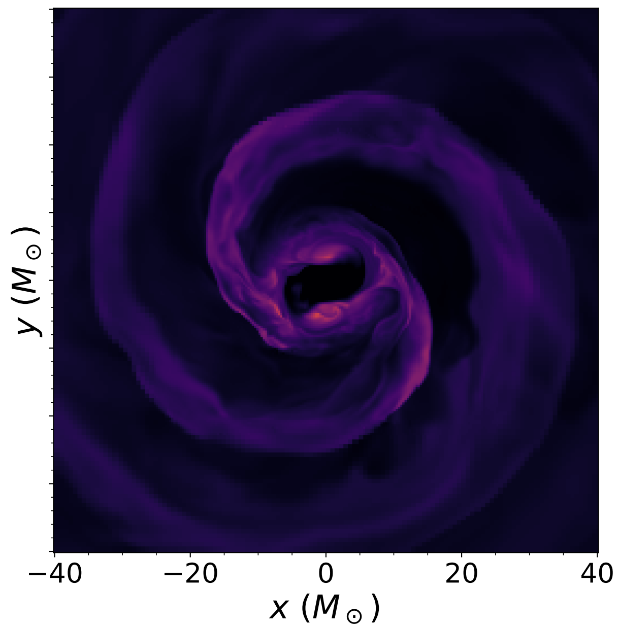
EOS-V 1.3 M_{\odot} - 1.3 M_{\odot} t = t_{\text{mrg}} + 3 \text{ ms}
