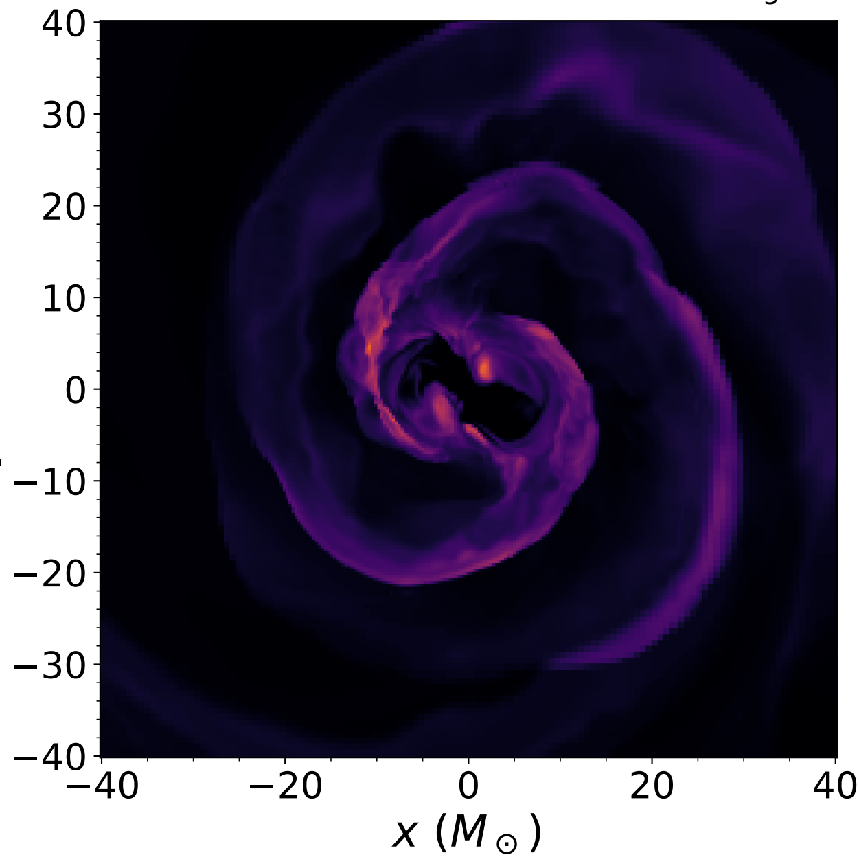
EOS-V 1.3 M_{\odot} - 1.3 M_{\odot} t = t_{\text{mrg}}
