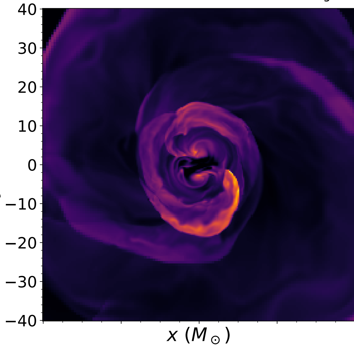
EOS-II 1.3 M_{\odot} - 1.3 M_{\odot} t = t_{\text{mrg}}
