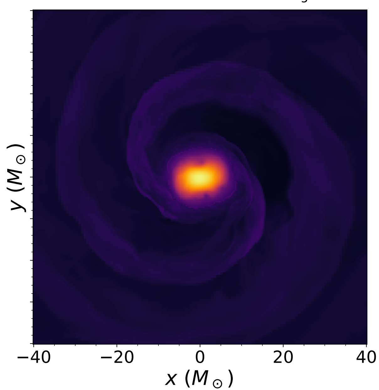
EOS-V 1.3 M_{\odot} - 1.3 M_{\odot} t = t_{\text{mrg}} + 3 \text{ ms}
