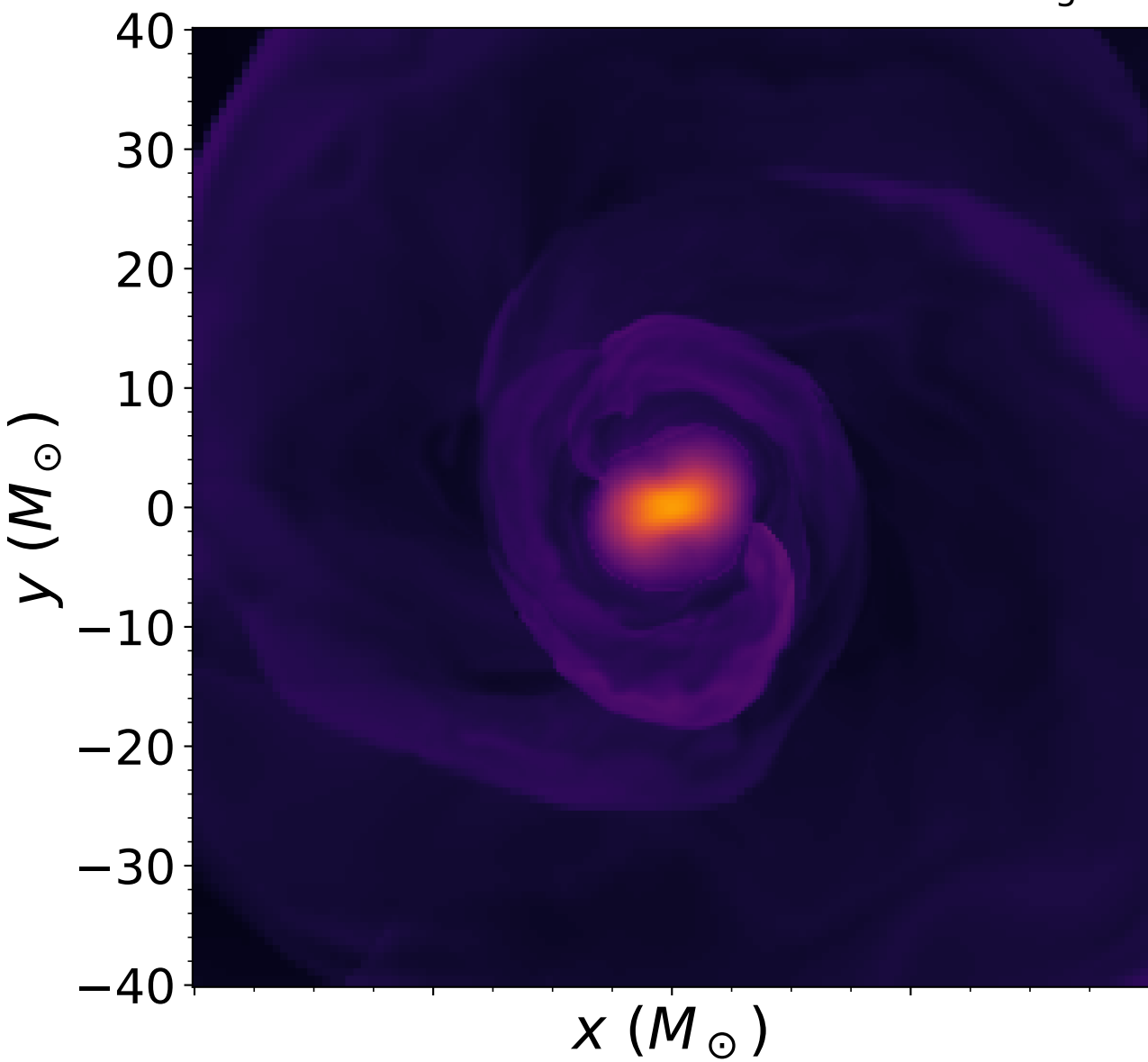
EOS-II 1.3 M_{\odot} - 1.3 M_{\odot} t = t_{\text{mrg}}
