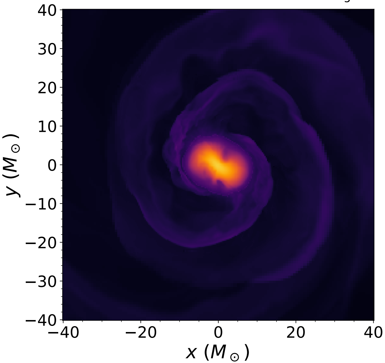
EOS-V 1.3 M_{\odot} - 1.3 M_{\odot} t = t_{\text{mrg}}
