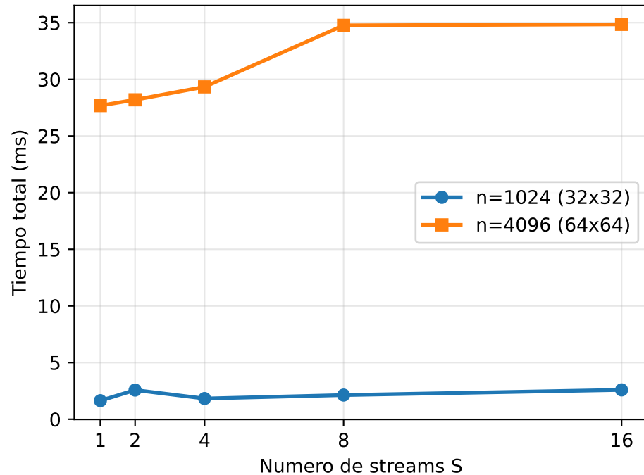
Tiempo total en funcion de S
