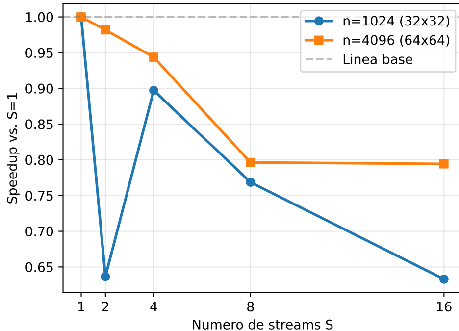
Speedup en funcion de S
