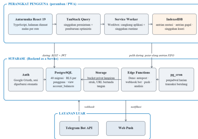
Gambar 1. Arsitektur sistem Tracr
