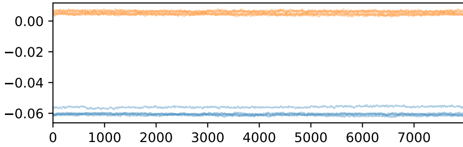
gamma_sheer_1
