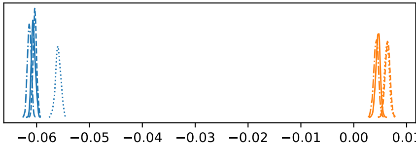
gamma_sheer_1
