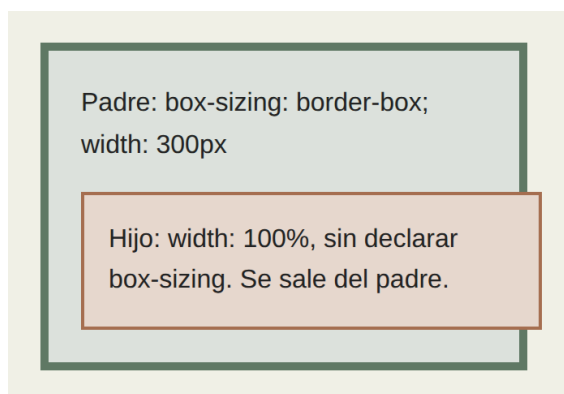
Figura 3. El hijo (284px) se sale de su padre border-box (300px) porque box-sizing no se hereda.
