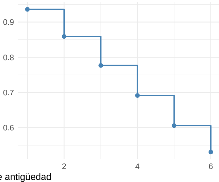
supervivencia S(t)
