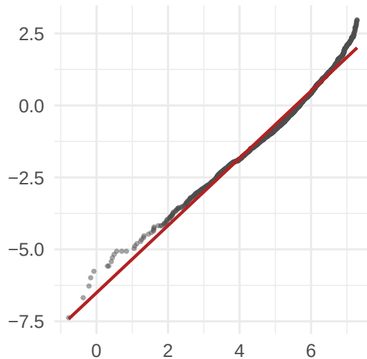
Log-logística: \text{logit}(1-S)
