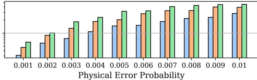
b) Chromobius
