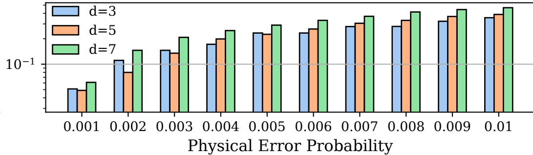
a) BP-OSD
