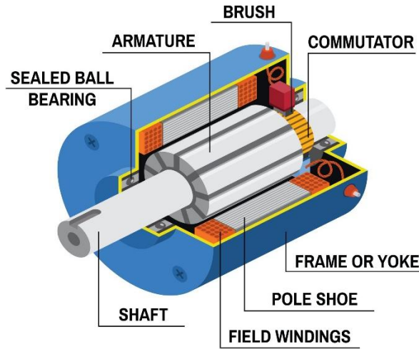
Şekil 11. DC motorun temel iç yapısı ve ana bileşenleri
