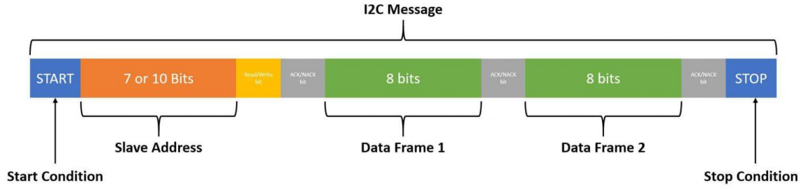
Şekil 6. I2C mesaj yapısında adres, okuma/yazma biti, ACK/NACK cevabı ve veri çerçeveleri
