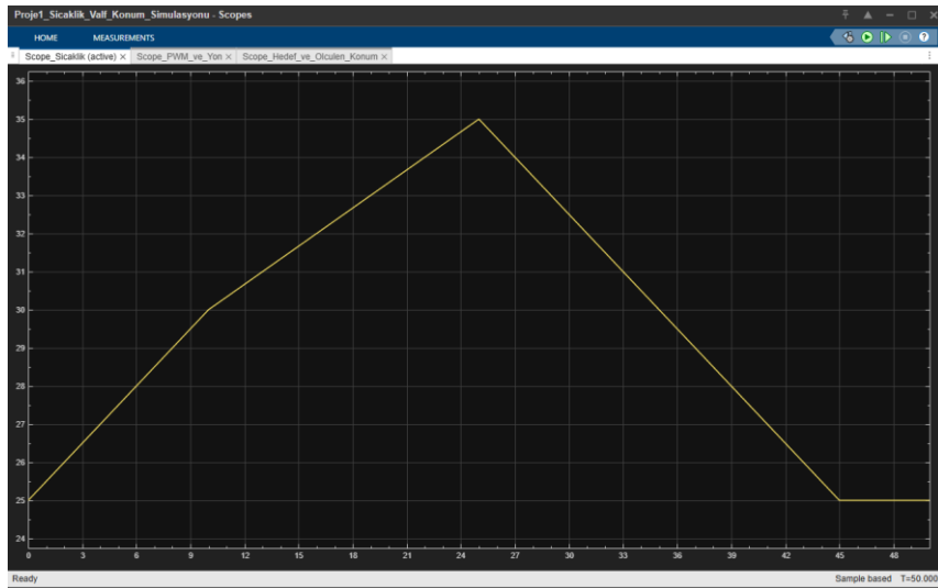
Şekil 34. Simülasyonda kullanılan sıcaklık giriş profili
