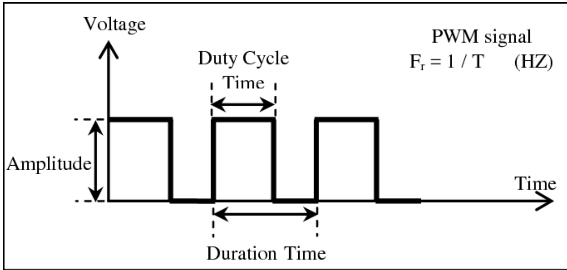
Şekil 19. PWM sinyalinin temel yapısı ve görev oranı gösterimi
