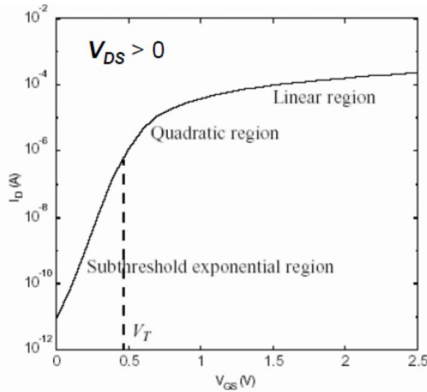
Şekil 21. MOSFET'in V_{GS} – I_D transfer karakteristiđi
