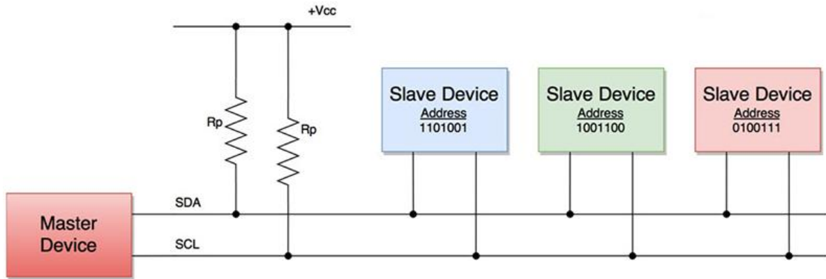
Şekil 7. I2C haberleşmesinde master-slave cihaz yapısı
