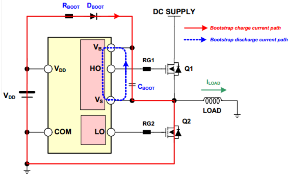
Şekil 26. Bootstrap devresi ile high-side MOSFET sürme mantığı
