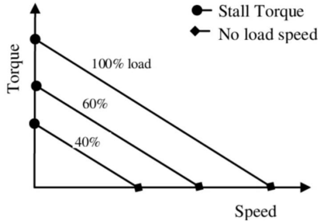
Şekil 15. DC motorun hız-moment karakteristiği
