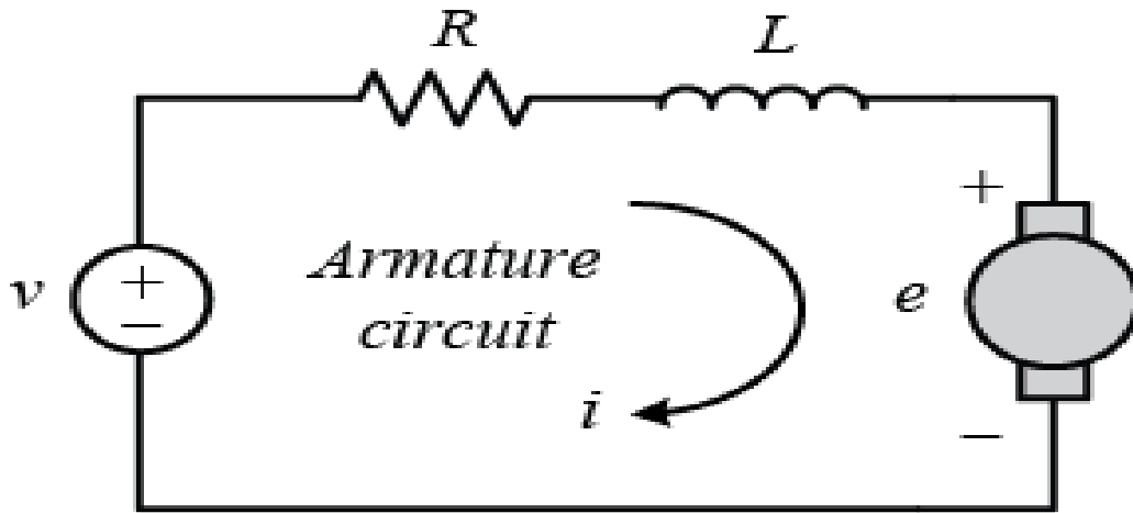
Şekil 13. DC motorun elektriksel eşdeğer devresi
