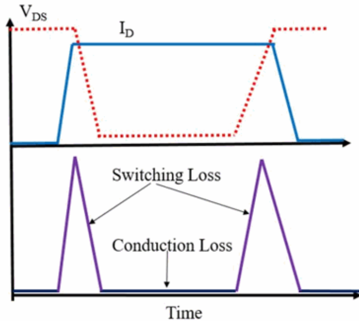
Şekil 23. MOSFET’te iletim ve anahtarlama kayıplarının zamana bağlı gösterimi
