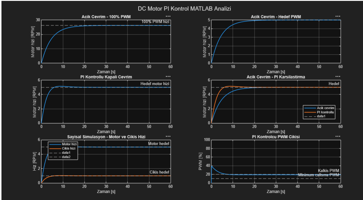
Şekil 37. Proje 2 kapsamında PI kontrollü düşük hız motor kontrolü MATLAB analiz sonuçları
