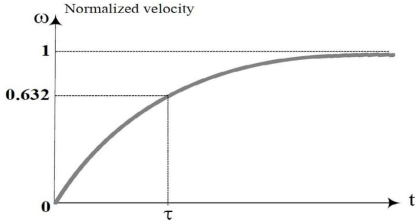
Şekil 17. Birinci dereceden yaklaşık DC motor hız modelinde normalize edilmiş hız cevabı ve zaman sabiti
