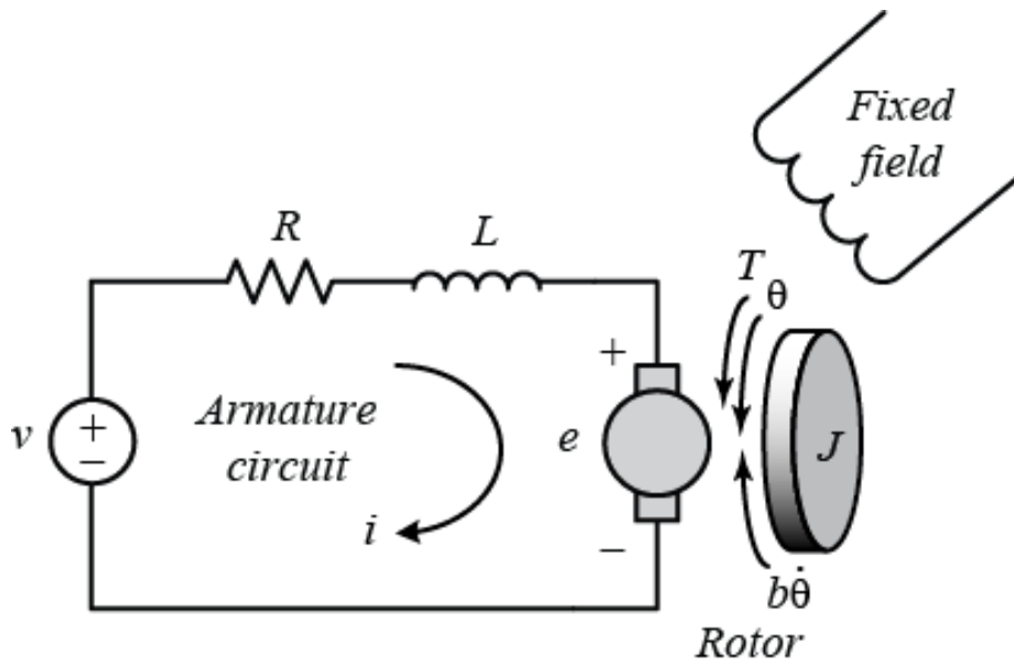
Şekil 14. DC motorun elektriksel eşdeğer devresi ve mekanik yük ile ilişkisi
