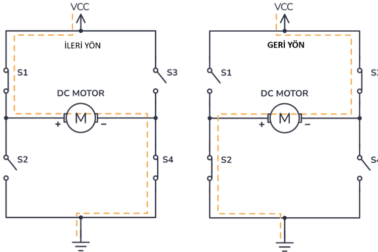
Şekil 24. H-köprüsü motor sürücü yapısında ileri ve geri yön akım yolları
