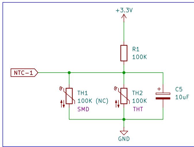
NTC Ambient Temp Sensor (Room)
