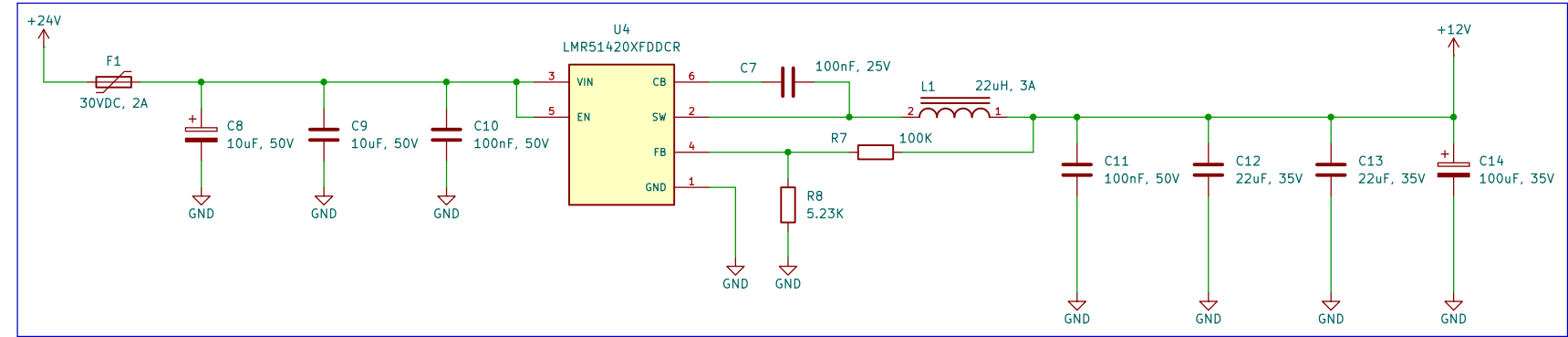
12V, 2A Buck Converter (PWM Fan Power)
