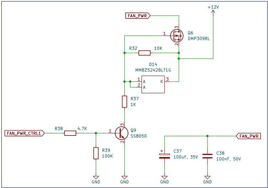
12VDC PWM Fan Power Control
