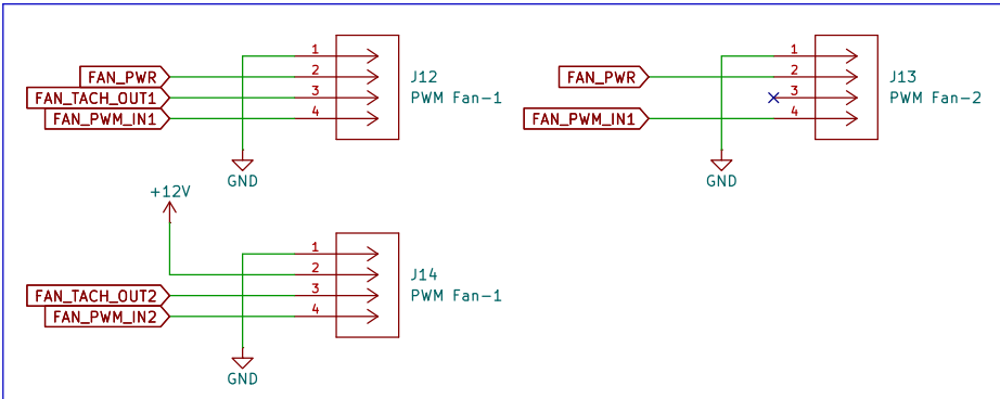
12VDC PWM Fan Connectors
