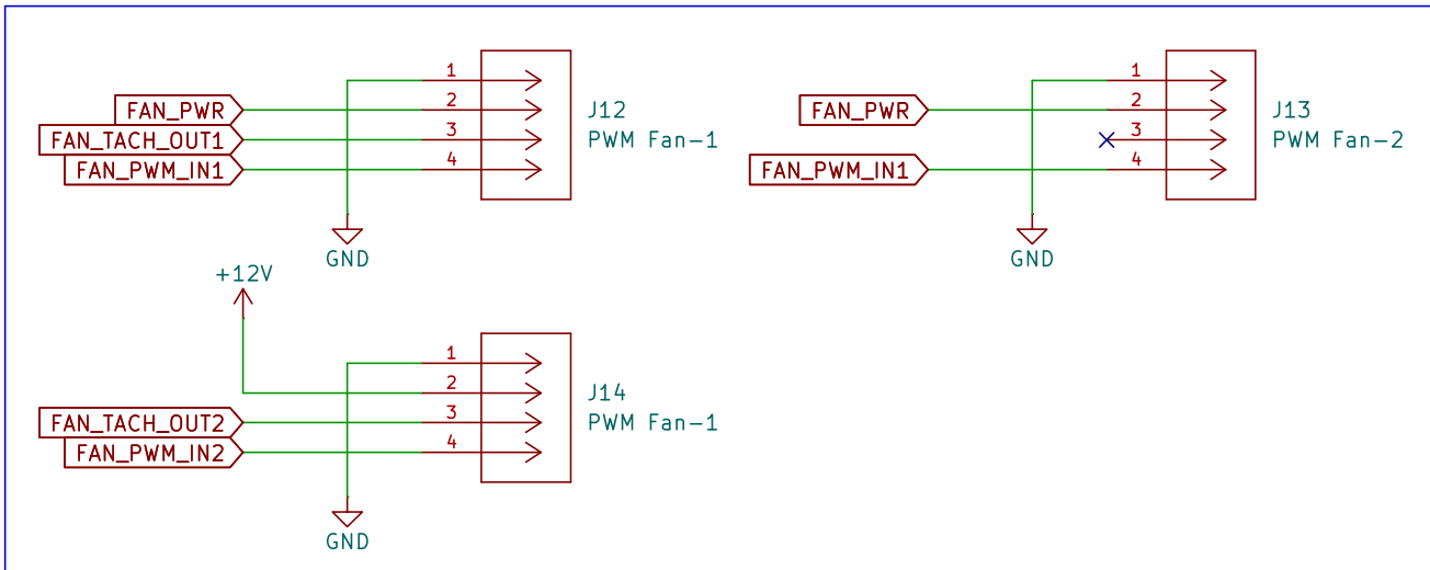
12VDC PWM Fan Connectors
