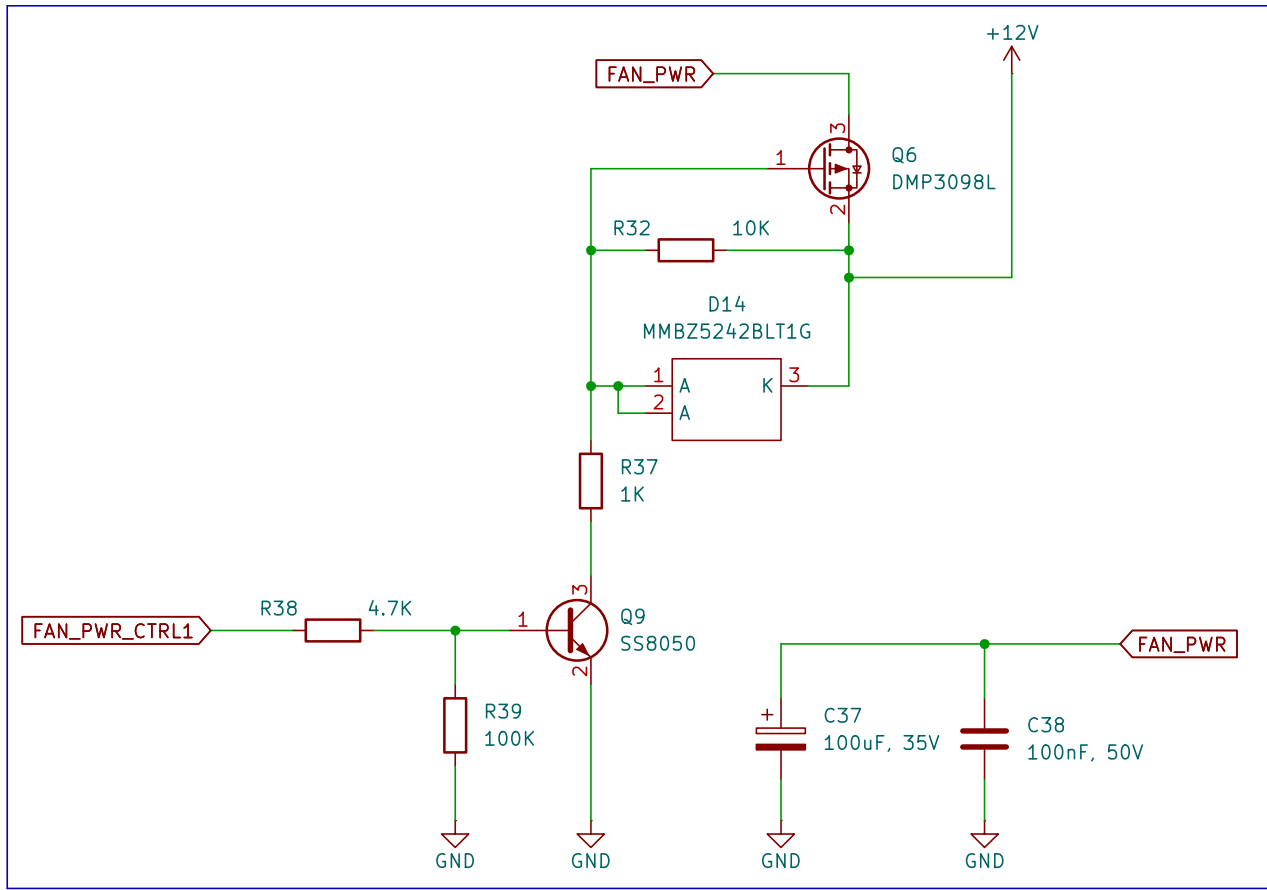
12VDC PWM Fan Power Control
