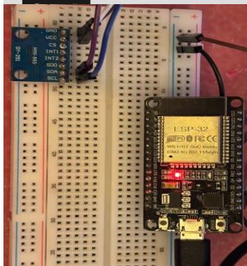
Abb. 2: Realer Versuchsaufbau — ESP32 mit ADXL345 (GY-291 Modul) auf Breadboard Verschaltung: VCC → 3.3V | GND → GND | SDA → GPIO 21 | SCL → GPIO 22
