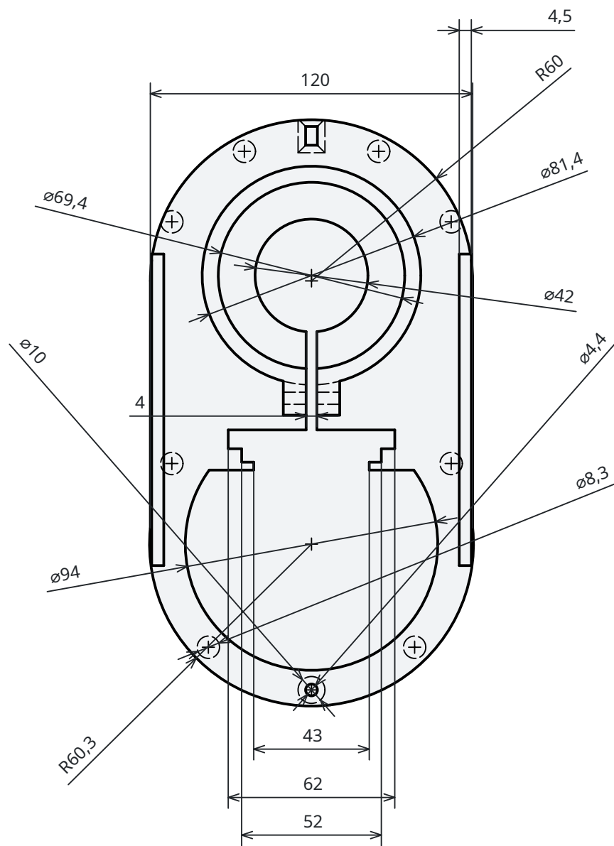
Dessus — le nez du conduit vers le bas
