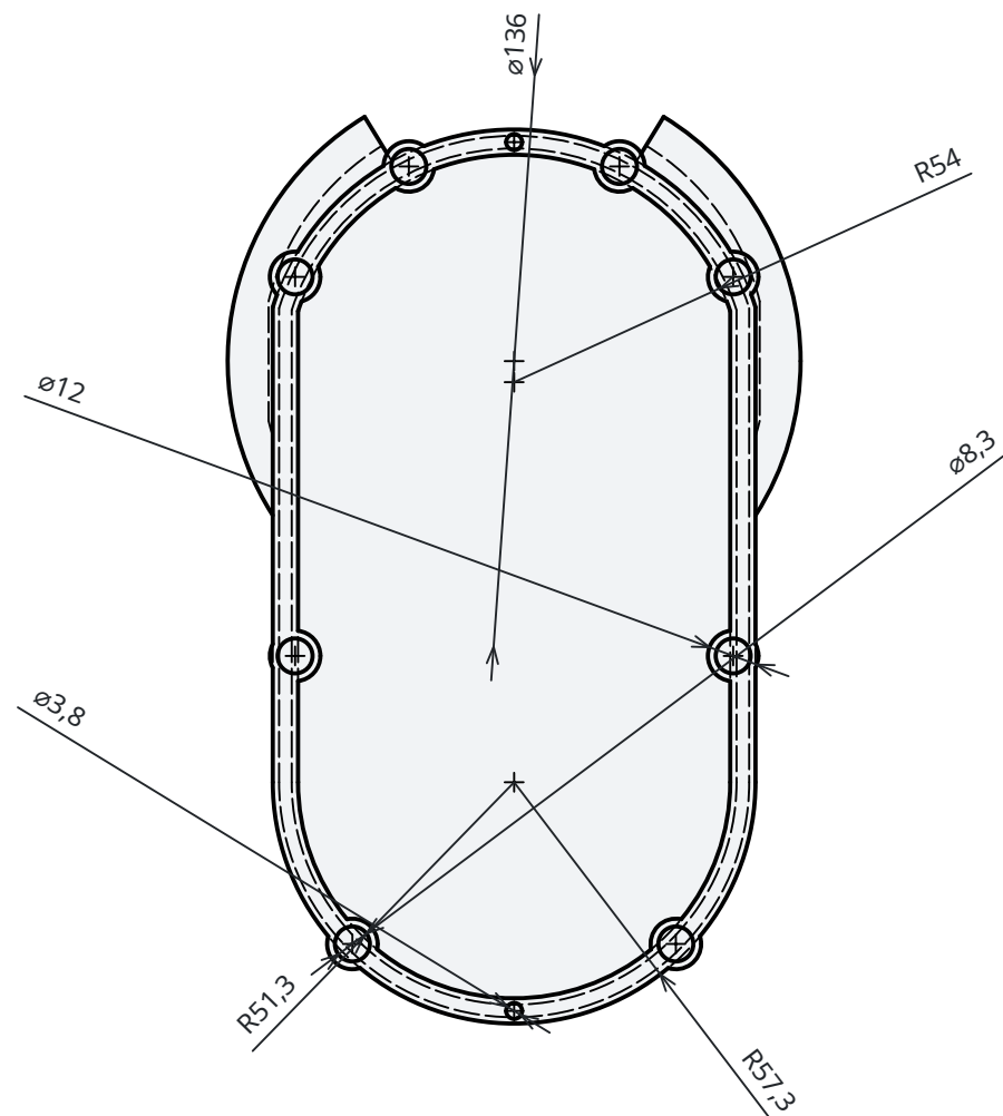
Dessus — la flasque à aimants
