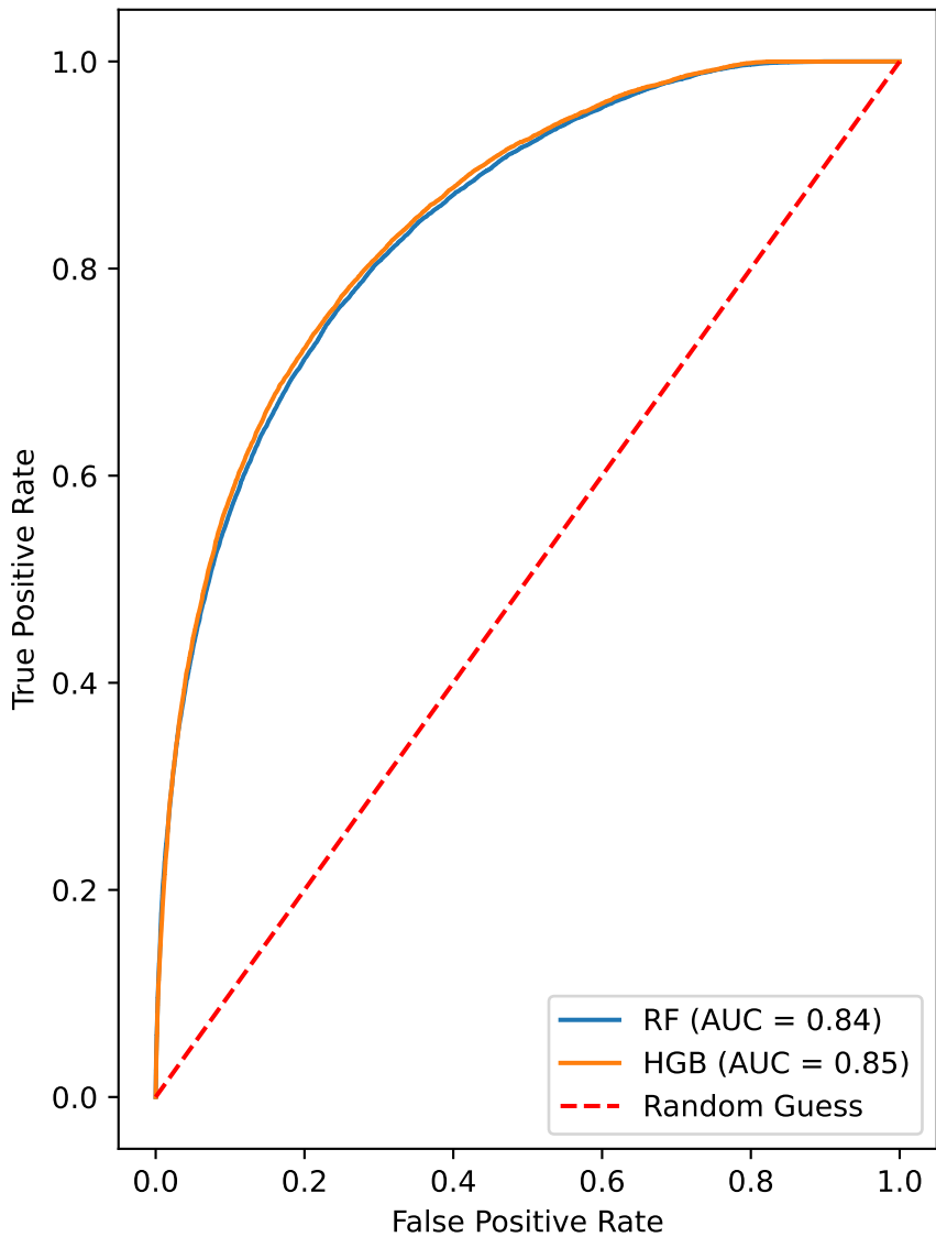
ROC courbes pour deux modèles
