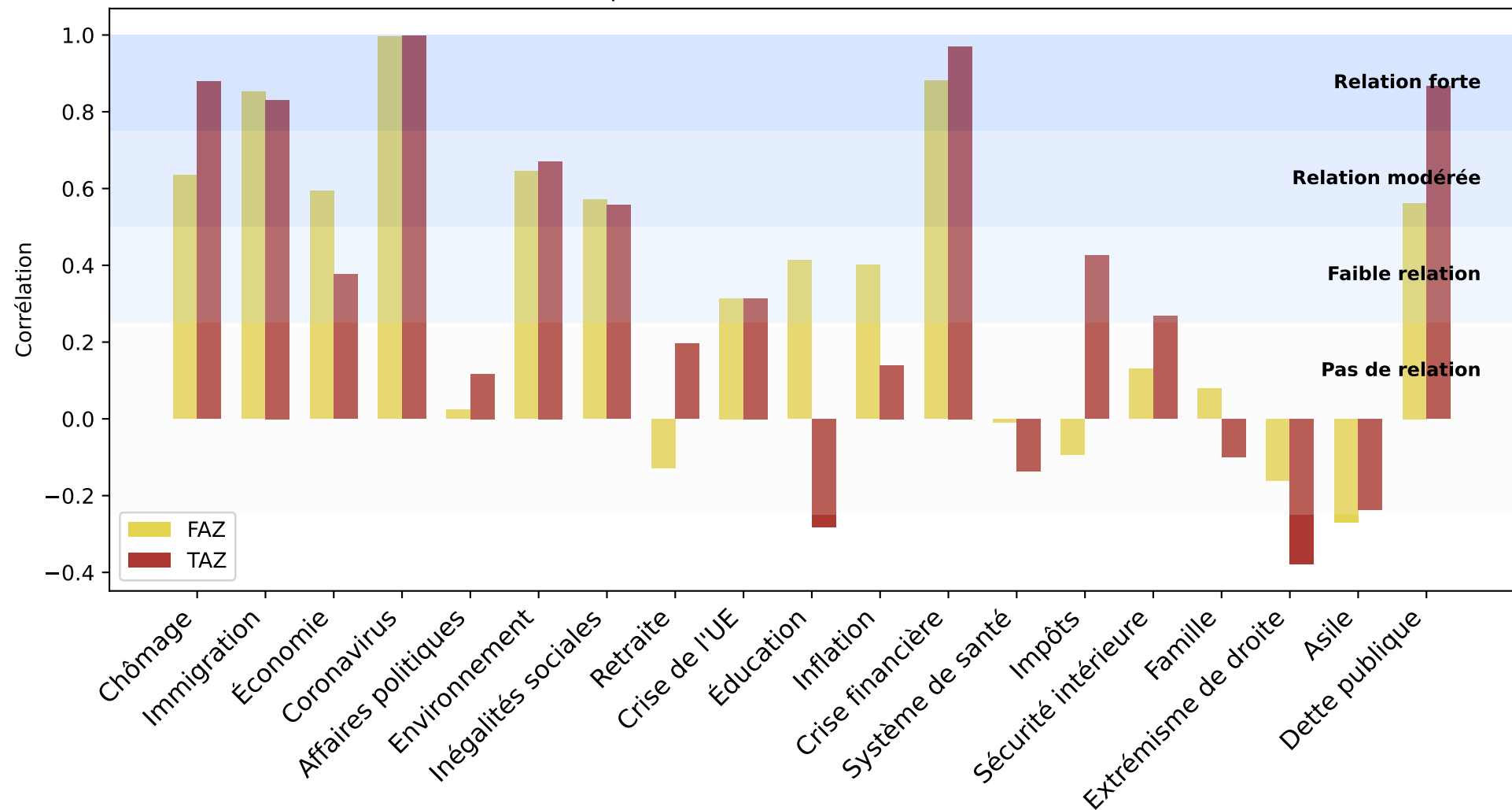
Comparaison des matrices de corrélation
