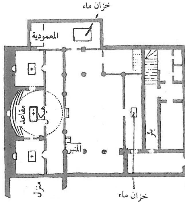
شكل رقم ٨: رسم تخطيطى لكنيسة الأنبا شنودة.
