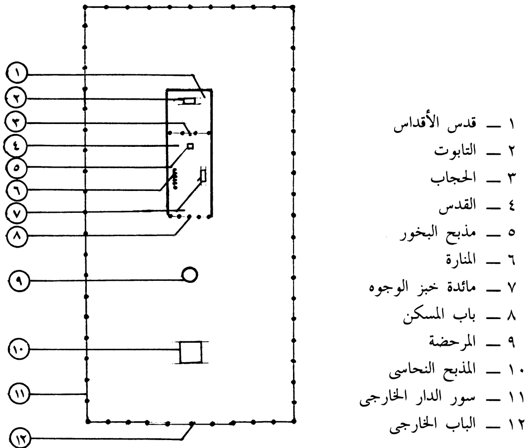
رسم خطى للمسكن والدار الخارجية بكل مشماتهما
