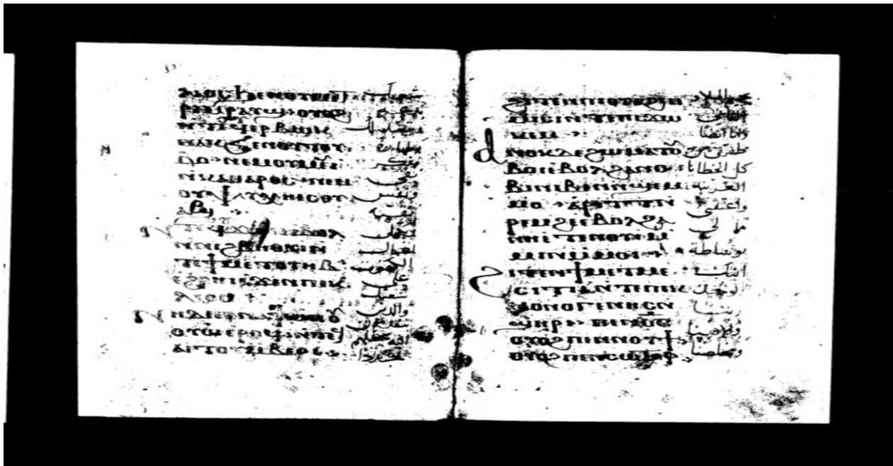
Codex ( B ) :
