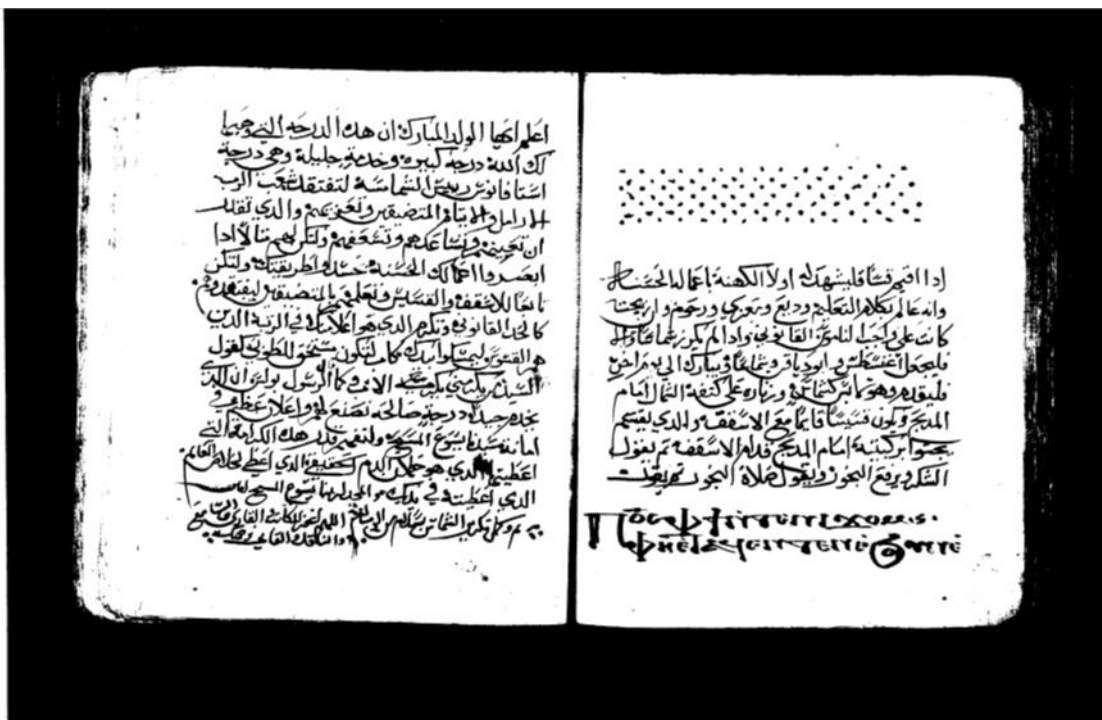
Codex ( I )
