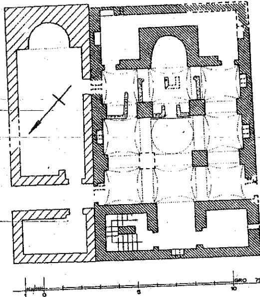
24 Die Kirche von Gindinarri
