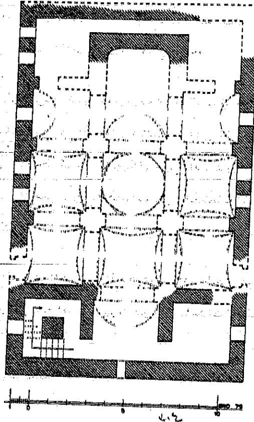
Abb. 68. Die Kirche von Fakhridib
