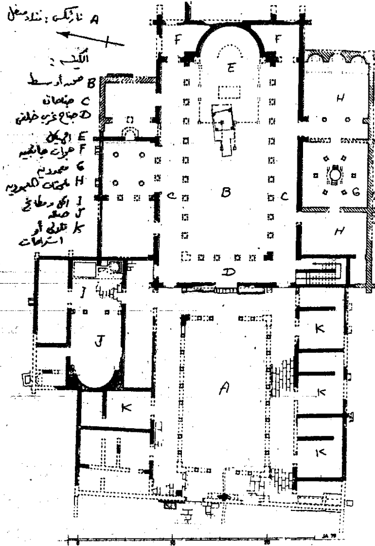
الكنيسة الشمالية بأبي مينا
