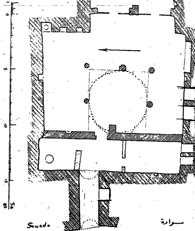
دير أباهور بدير سواده شرق المنيا
