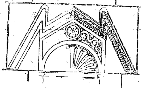
Fig. 35. Dér el Abiad. Head of niche.
