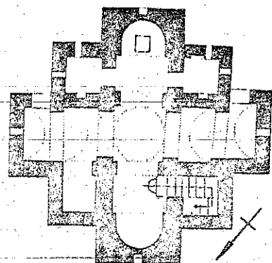
Die Engelskirche von Tamit. Grundriß und Schnitt
