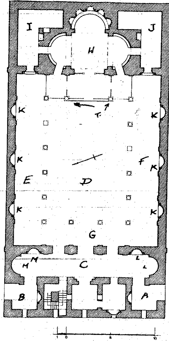
كنيسة داخل معبد هاتور بدندره
