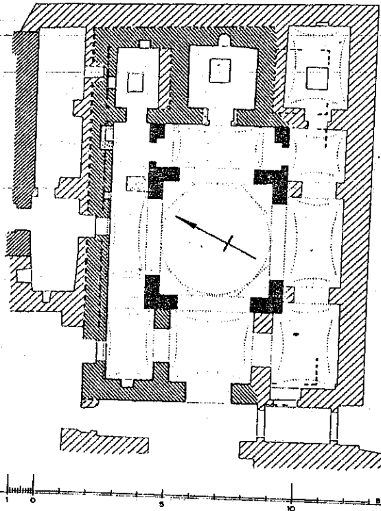
Die Kirche von Dair al-Fahūrī bei Aṣṣūn (nach G. Castel)
