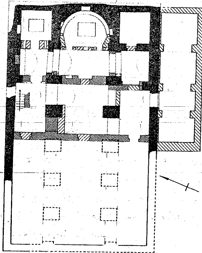
Die Georgskirche von Dair al-Magma bei Nuqada
