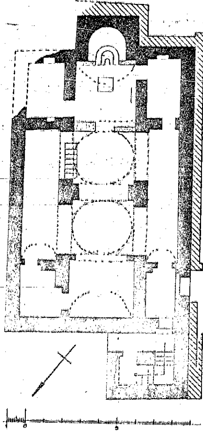
Die 'Basilika' von Tamt (Nubien)
