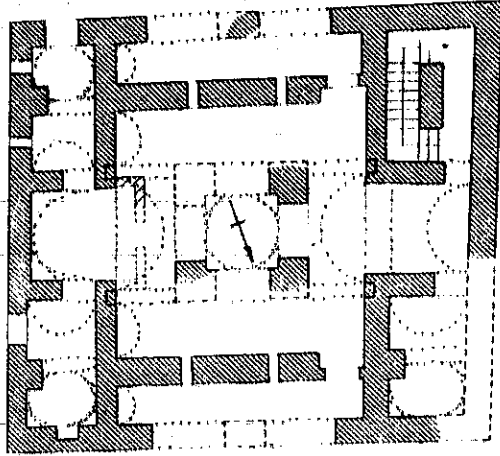
Die Wüstenkirche von Adindān, Gr
