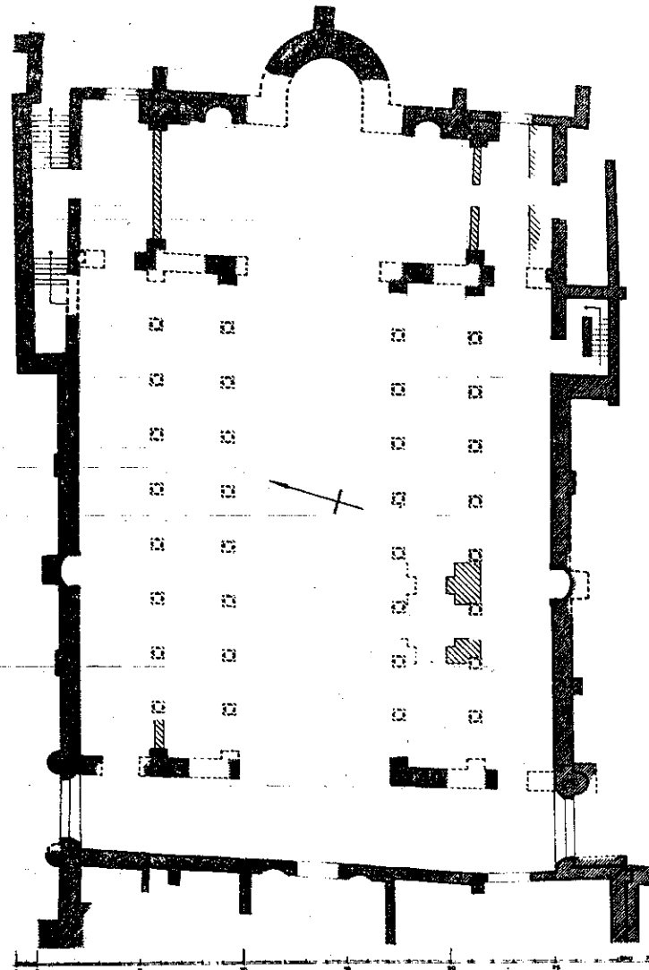
كنيسة المدفن في القرن الثامن
