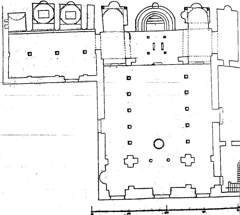
الست بربارة بمصر القديمة.
