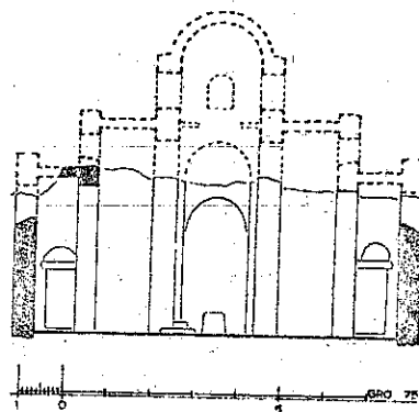
Die Engelskirche von Tamit. Grundriß und Schnitt
