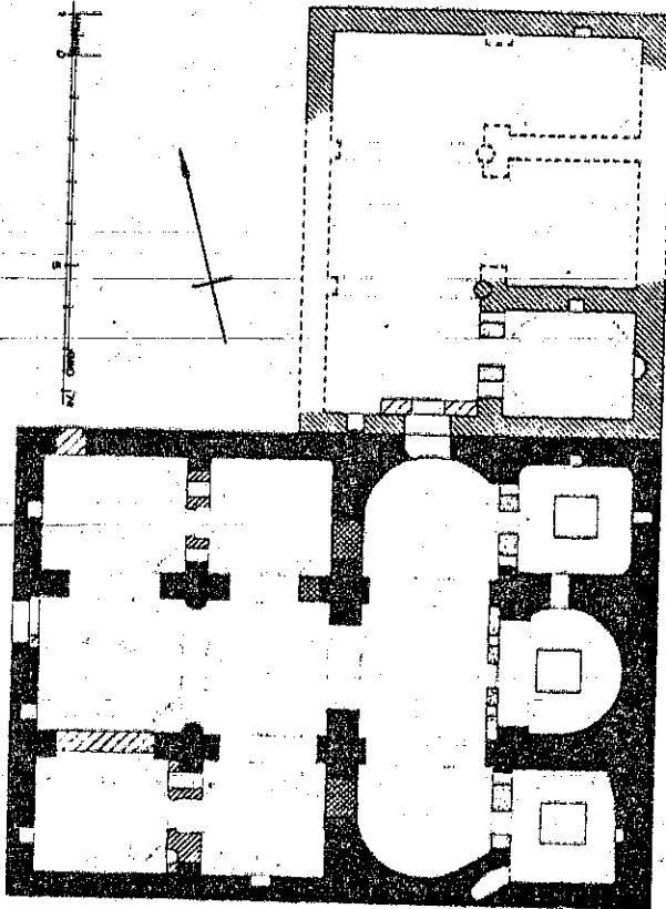
Die beiden Kirchen von Dar al-Malak Milbeti bei Gnamla
