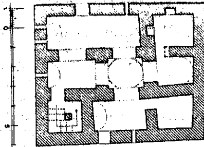
Abb. 72. Die Zentralkirche von Sirra. Unter- und Obergeschoss
