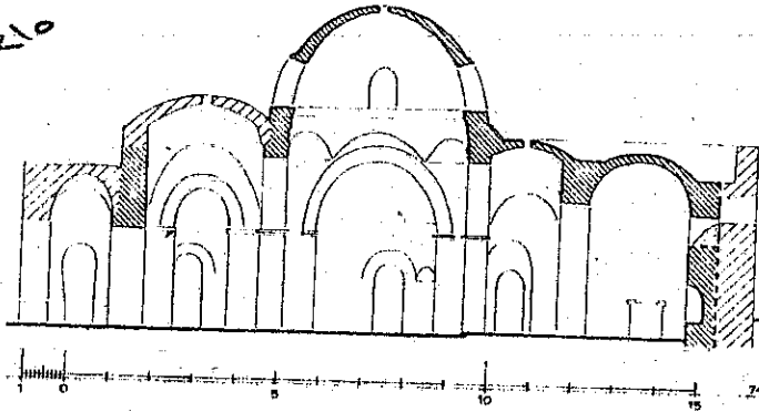
Längsschnitt durch die Kirche von Dair al-Fahūrī (nach G. Castel)
