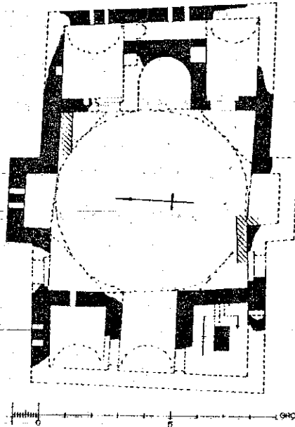
abb. 20. Grundriß der Kuppelkirche von Kulb
