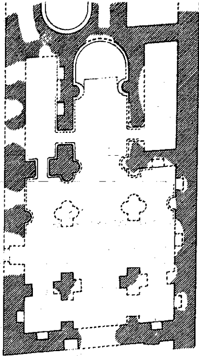
كنائس حلوان الأثرية ١
