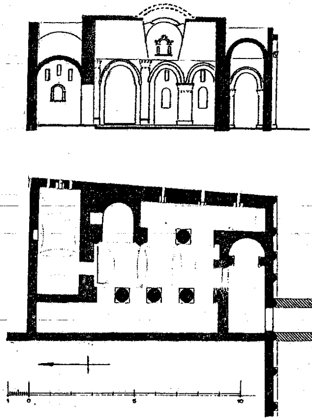
Die Kapelle 25 von al-Bagawät. Grundriß und Schnitt.
