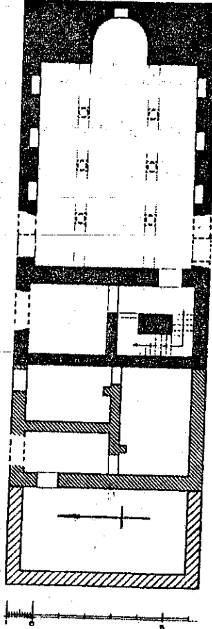
Die Kirche von Sitt Gasma in Nubien
