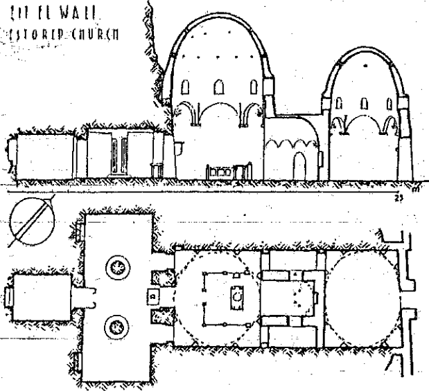
كنيسة بيت الوالى بالنوبة
