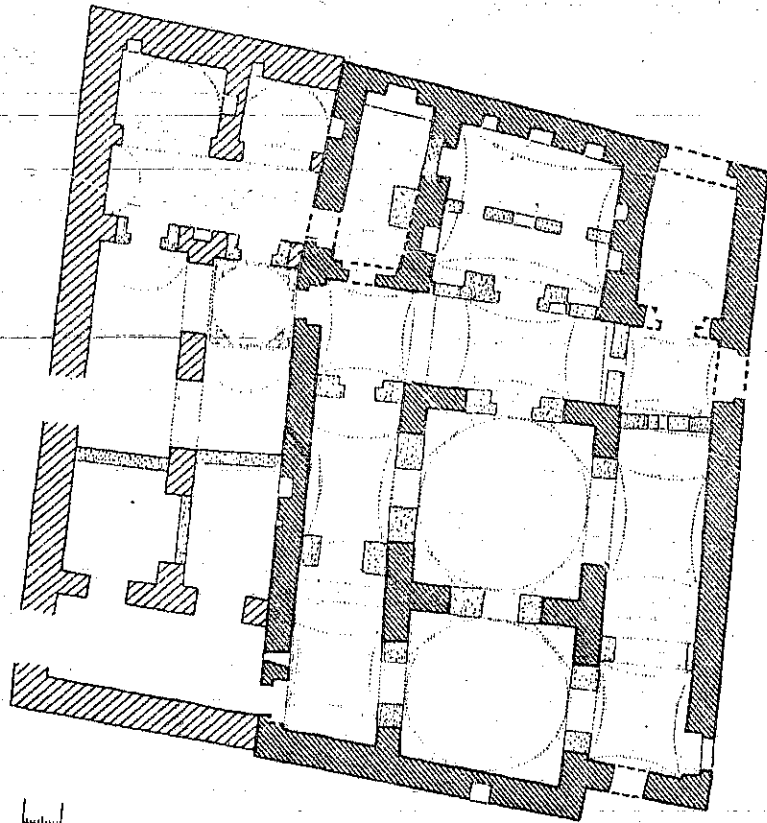
1. Grundriß von Dair aš-Šuhadā' bei Isnā (nach G. Castel)
