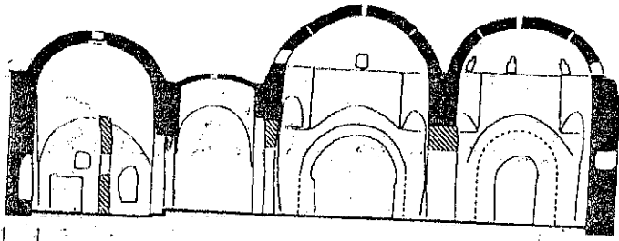
Abb. 9 Längsschnitt durch die Hauptkirche von Dair aš-Šuhadā'
