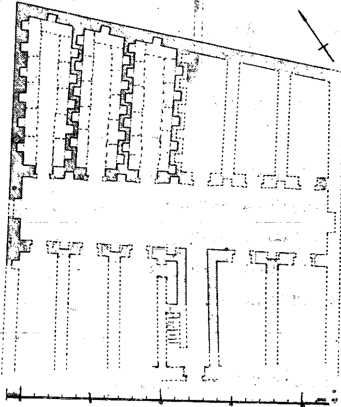
Unterkunftsbau eines Klosters nördlich von Dair Abū Hinnis (Grabung A. R. Abdel Tawab).
