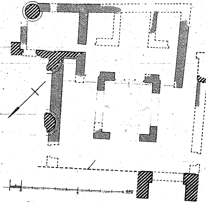
Die Kirche im Pnaos des Chnumtempels von Elephantine
