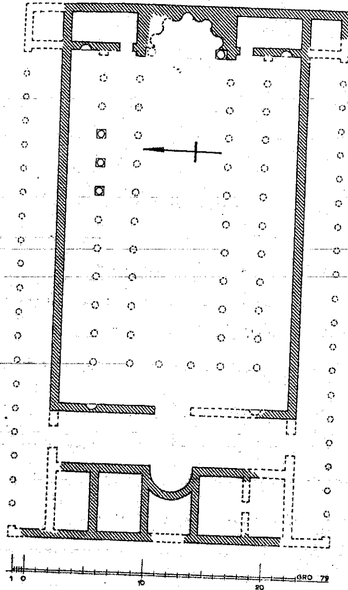
e Basilika von Armant. Neuzeichnung nach R. Pococke (1743), E. Joinard (1798-1801) und J. Burton (1830-1835).
