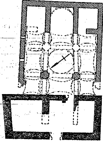
Kirche von Madiq bei Garf Husain
