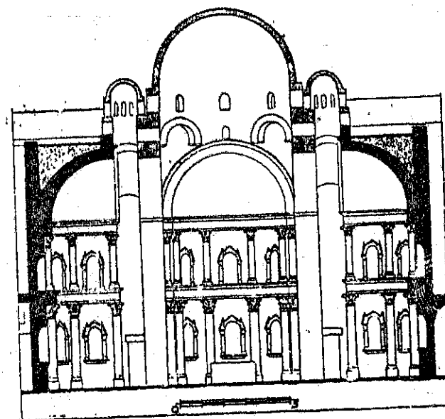
قطاع بكنيسة الالبا شتوده (الدير الابيض) قرب سوهاج
