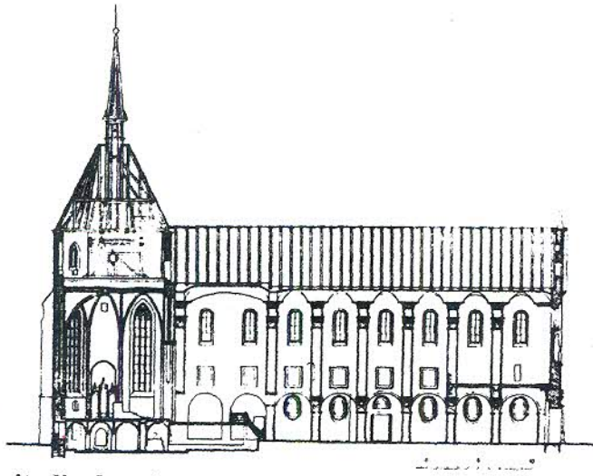
Longitudinal section of the Church of St. Verena in Zurzach A. Reinle, Die Heilige Verena von Zurzach, Basel 1948
