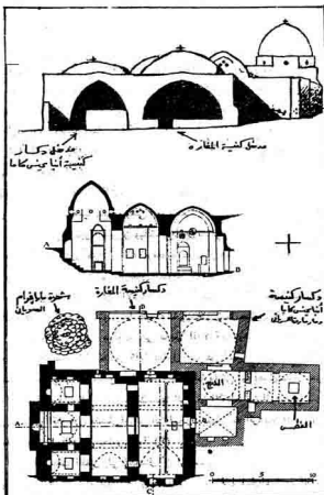
الرسم المعماري لكنيسة المغارة وكنيسة أنبا يحيى كاما ومار ماروتا السيراني التي تقع في الجزء الغربي من كنيسة المغارة .
