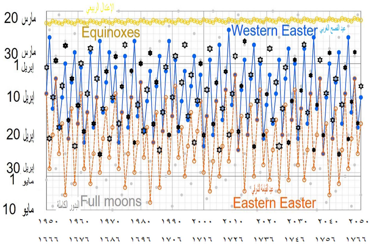
شكل ١ - الإعتدالات: الدوائر الصفراء - تواريخ عيد الفصح الغربي: دوائر مغلقة زرقاء - أقمار كاملة: دوائر رمادية مغلقة -
