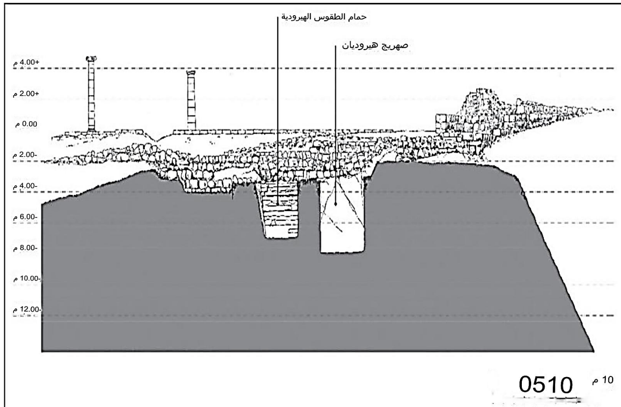
22. مقطع عرضي للحمام الطقسي الهيرودي والصهرج الهيرودي.
