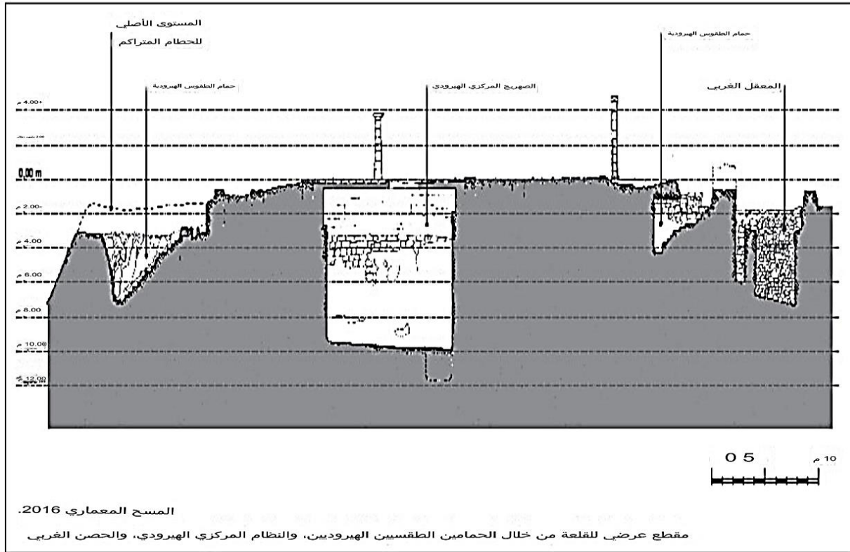
21. مقطع عرضي للقلعة، عبر الحمامات الهيرودية، والصهرج الهيرودي، والحصن الغربى.
