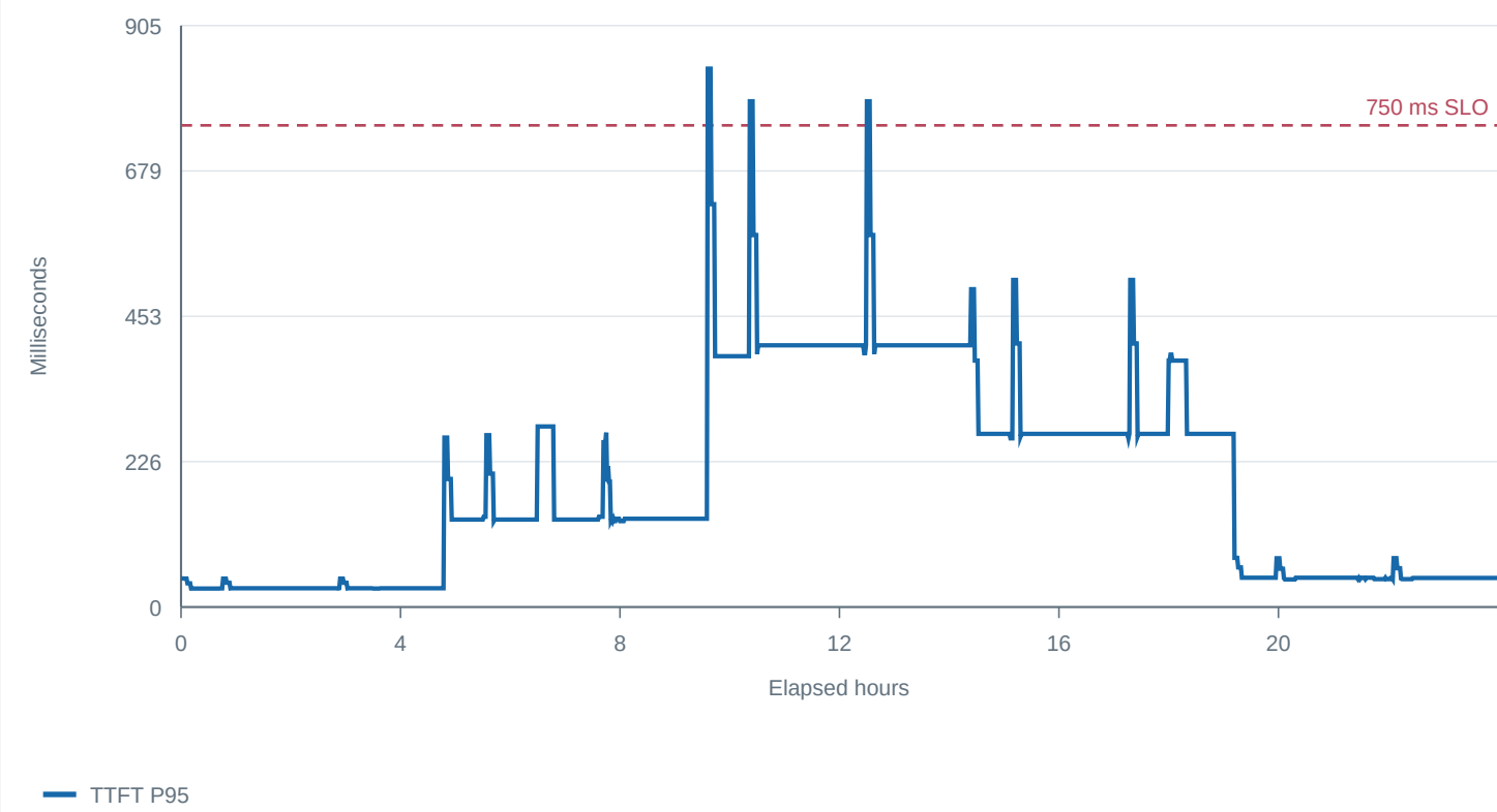
TTFT P95
