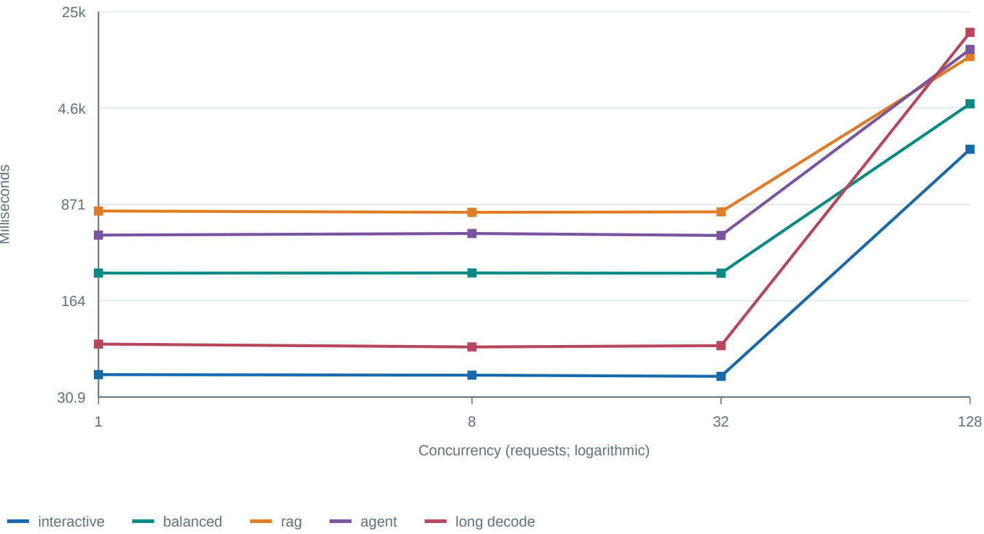
Mean run P95 TTFT
